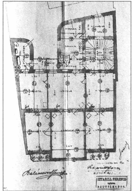
Casa Balássovits Planul etajului curent
