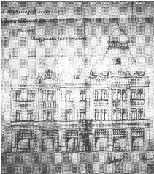
Casa Andrényi, fațada dinspre Piața 1 Decembrie, proiect din 1913 și imagine actuală
