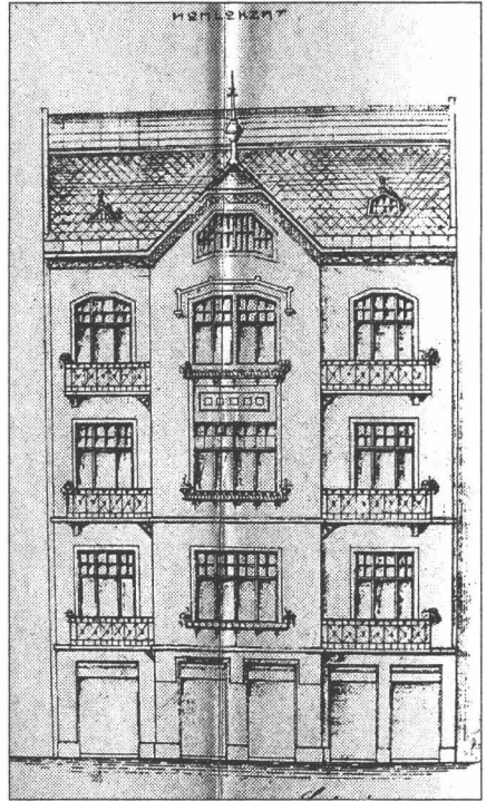
Casa Balássovits Al doilea proiect de fațadă
