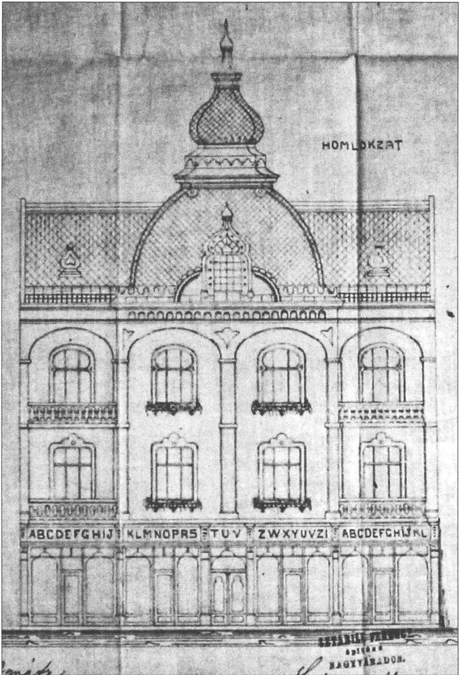
Imobilul Jungreis Ignác și Jungreis Antal, proiectul pentru fațada dispere actuala str. Crinului, 1912
