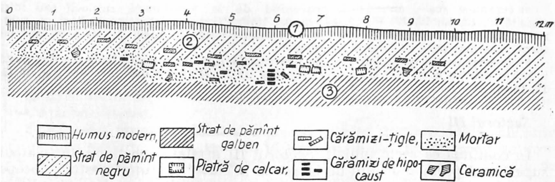
Fig. 18. Profilul clădirii romane cu hipocaust
