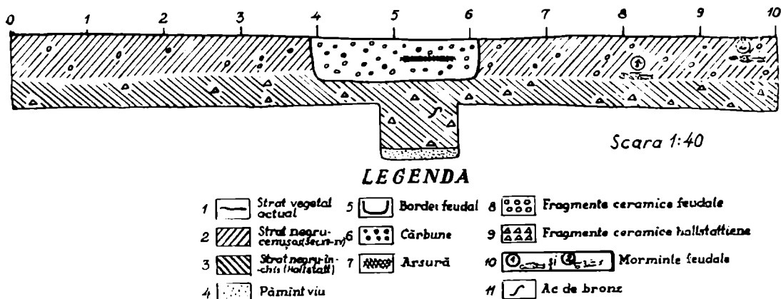
Fig. 2. Profilul secțiunii a III-a de la Sopor – Iacobeni.
