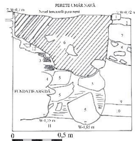
Fig. 32. S2. Profil Vest
