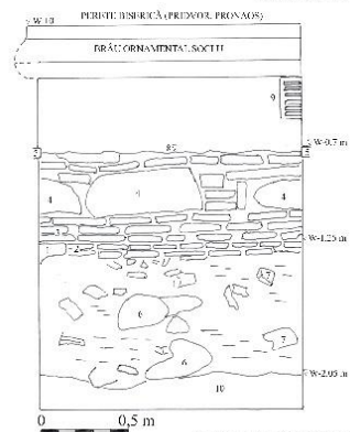
Fig. 24. S3a. Profil Nord
