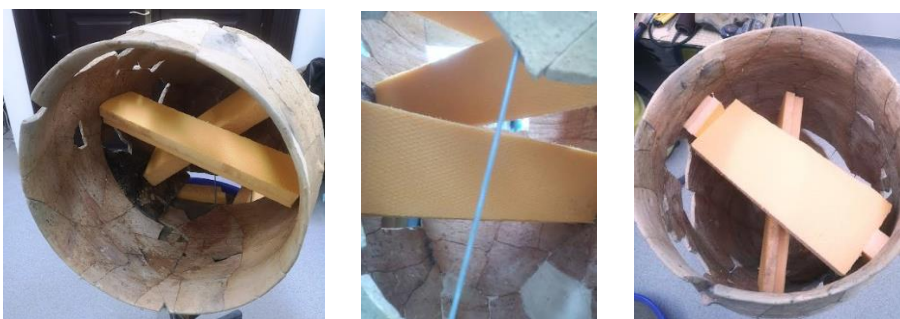
Fig. 7 – Montare elemente de susținere provizorii din polistiren extrudat
