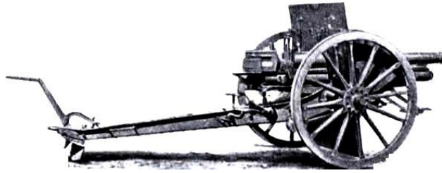
Fig. 3 Tun de câmp Skoda md. 1905 cal. 80 mm
