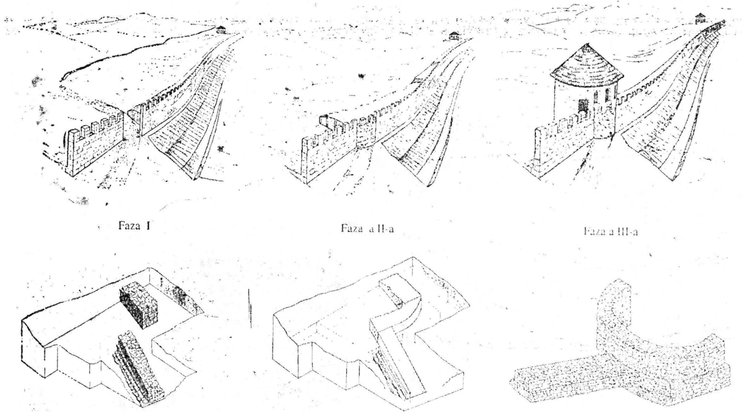
Fig. 4. Dealul Vișinal (în pădure); poarta de acces în provincia Dacia cu reconstituirea desenată a celor 3 principale faze de construcție
