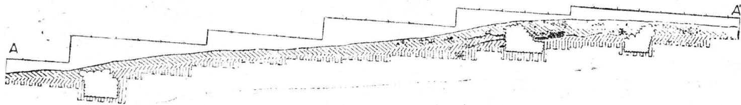
Fig. 3. Poarta Meseșană din zona Văii Făgiște de la Mirșid: a. Fotografie a porții Văii Făgiștii; b. Desenul zonei trecătorii din punctul Făgiște, cu zidul și cu amplasarea turnului din spatele zidului provinciei Dacia; c. Profilul secțiunii A—A' — prin zidul de apărare și turnul din spatele lui
