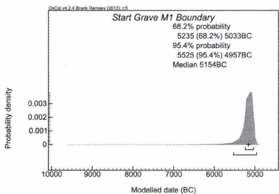
Fig. 4a. Distribuția probabilă a valorilor începutului fazei M1 obținută din modelarea datelor din Fig. 2
