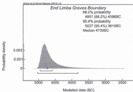
Fig. 3b. Distribuția probabilă a valorilor sfârșitului secvenței M1-M2 obținută din modelarea datelor din Fig. 2
