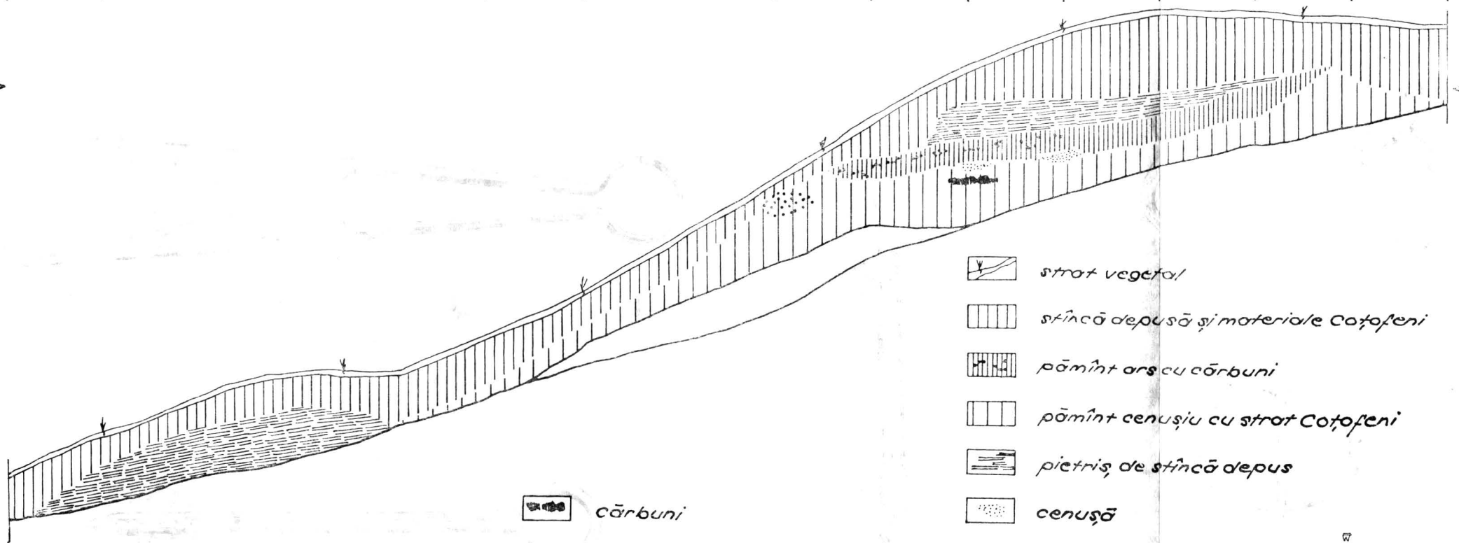
Planșa IV — Cetatea scurtă. Profilul peretelui de est al secțiunii VII.
