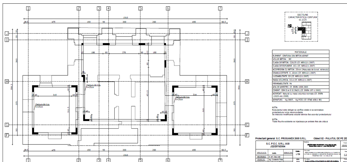
Fig. 2. Palatul de pe ziduri. Plan cofraj stâlpișori și centuri subsol.
