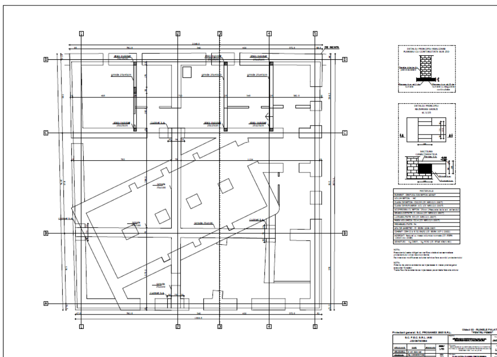
Fig. 3. Ruinele palatului „pentru femei”. Planul cofrajului planșeului de peste demisol.
