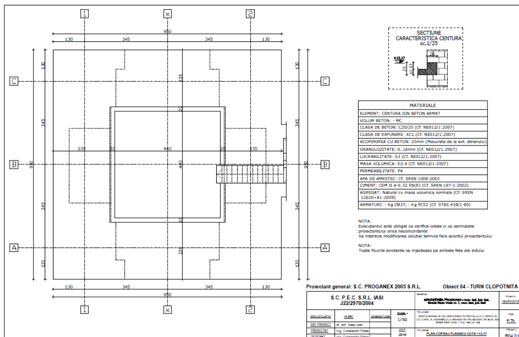
Fig. 4. Turnul clopotniță. Planul cofrajului pentru planșeu, cota +13,17m.
