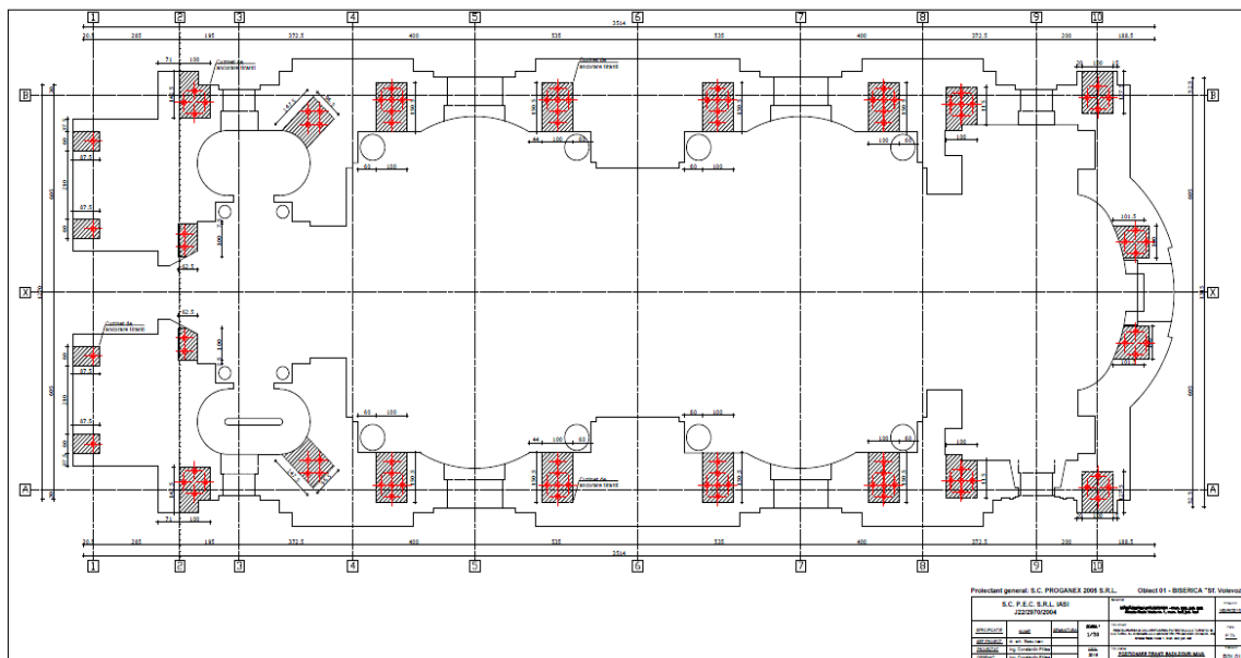
Fig. 1. Biserica. Poziționarea tiranților de la baza zidurilor navei (cota +0.00).
