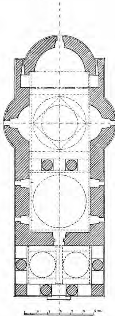
6. Biserica mănăstirii Aron-Vodă — Planul —
