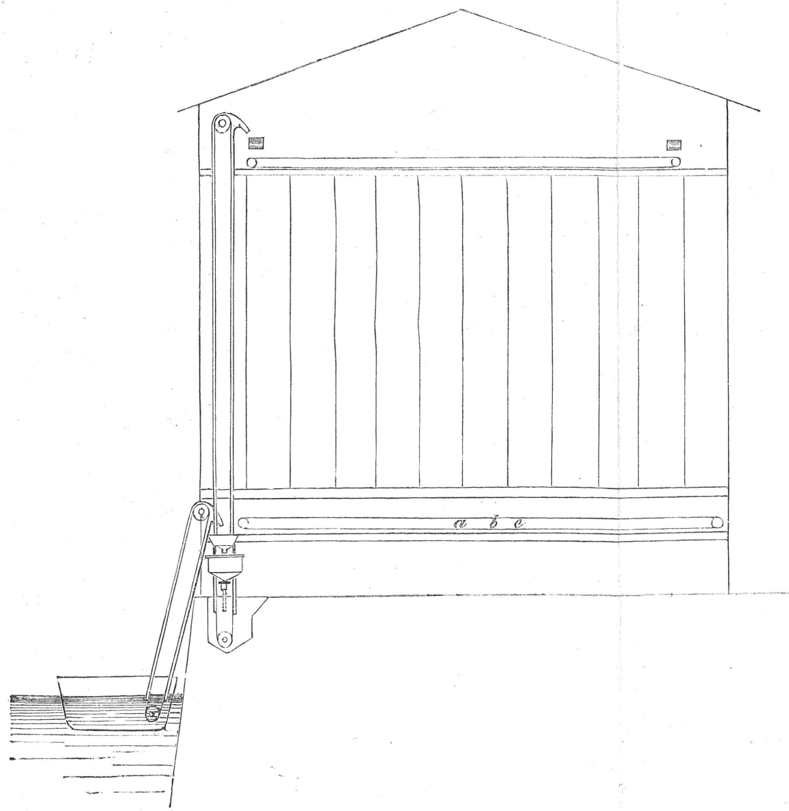
Secțiune prin a. b.
