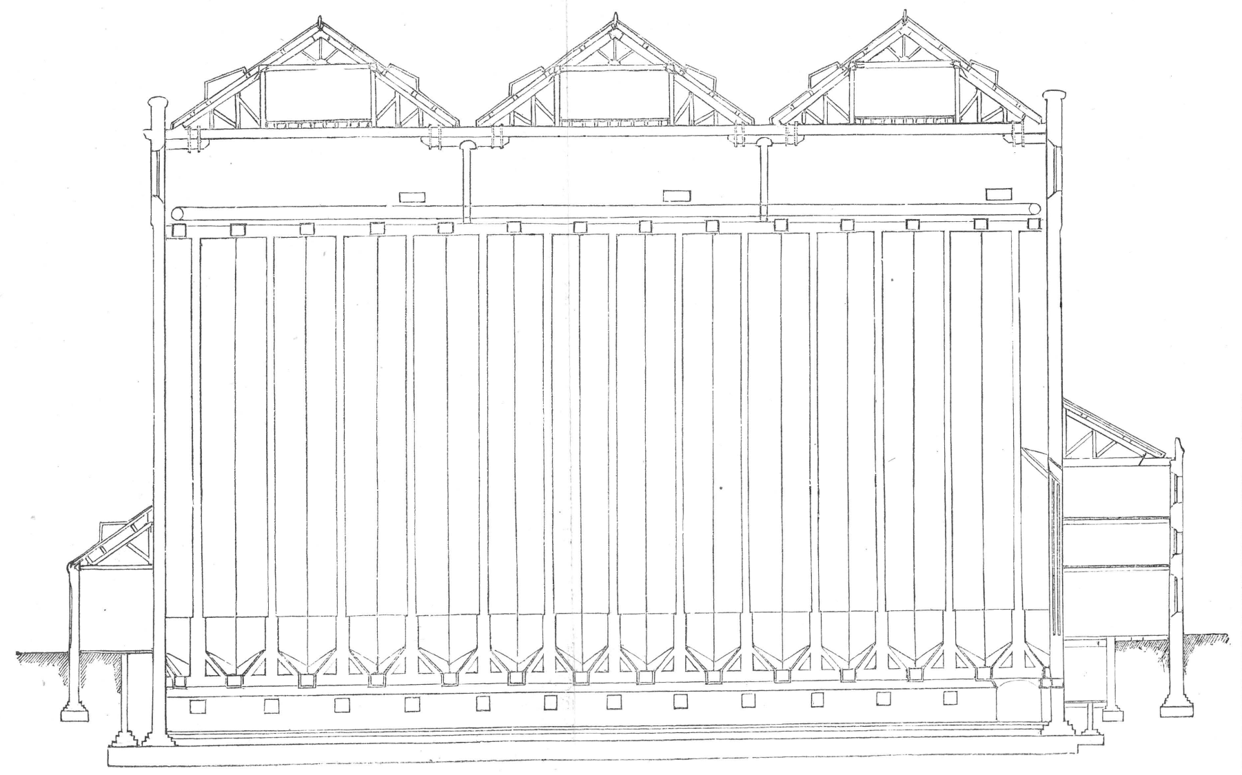
Seçione transversala
