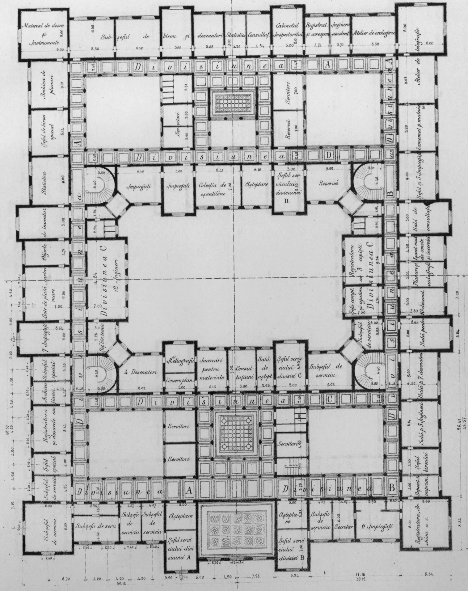
PLANUL ETAGIULUI II
