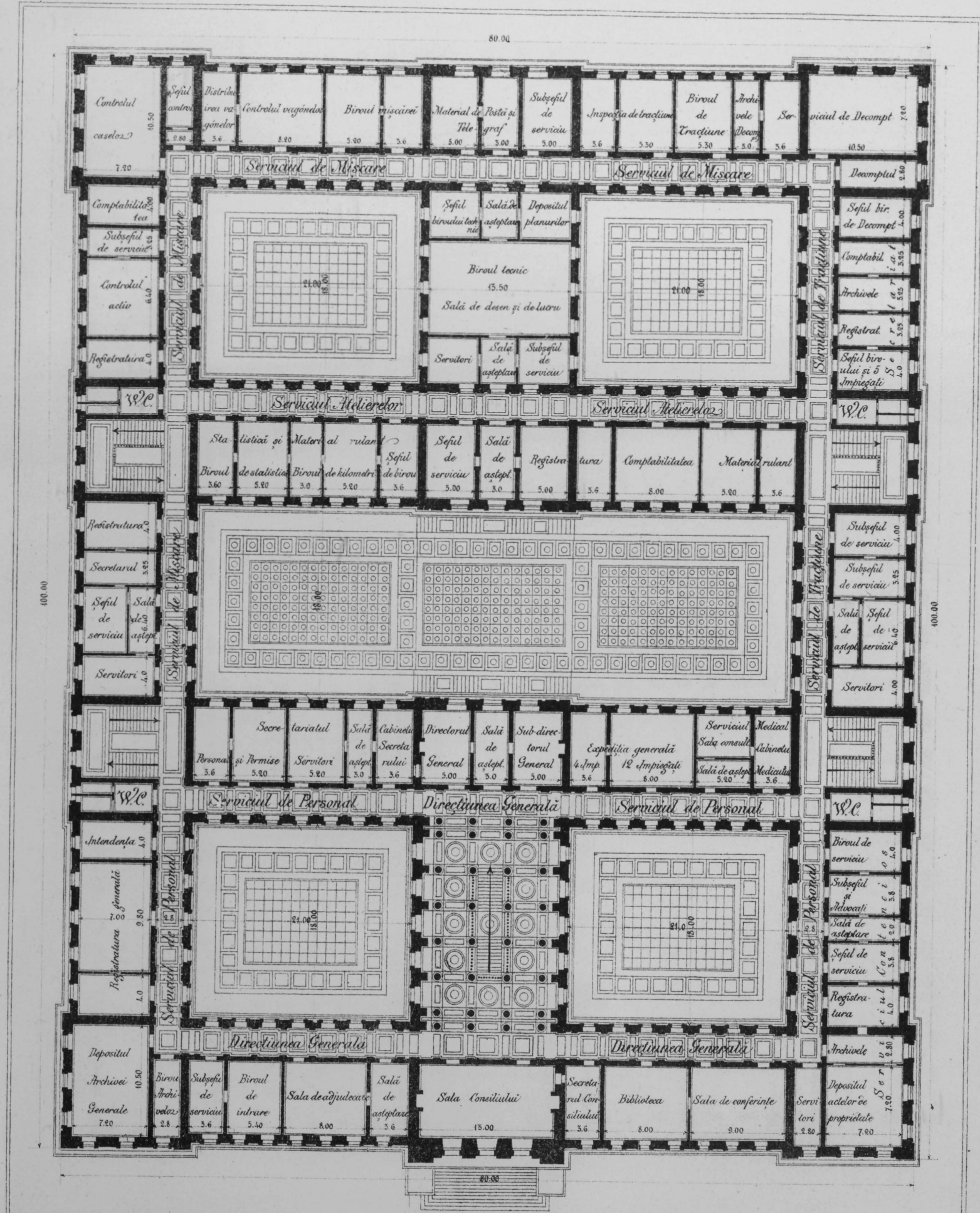
PLANUL ETAGIULUI I
