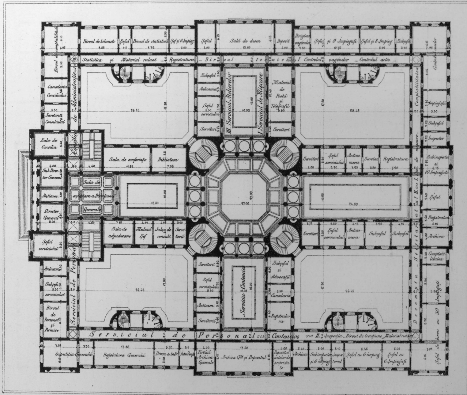
PLANUL ETAGIULUI I
