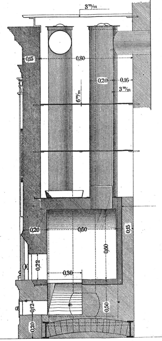
SECTIA CD
