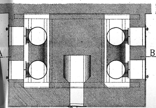
SECTIA EF
