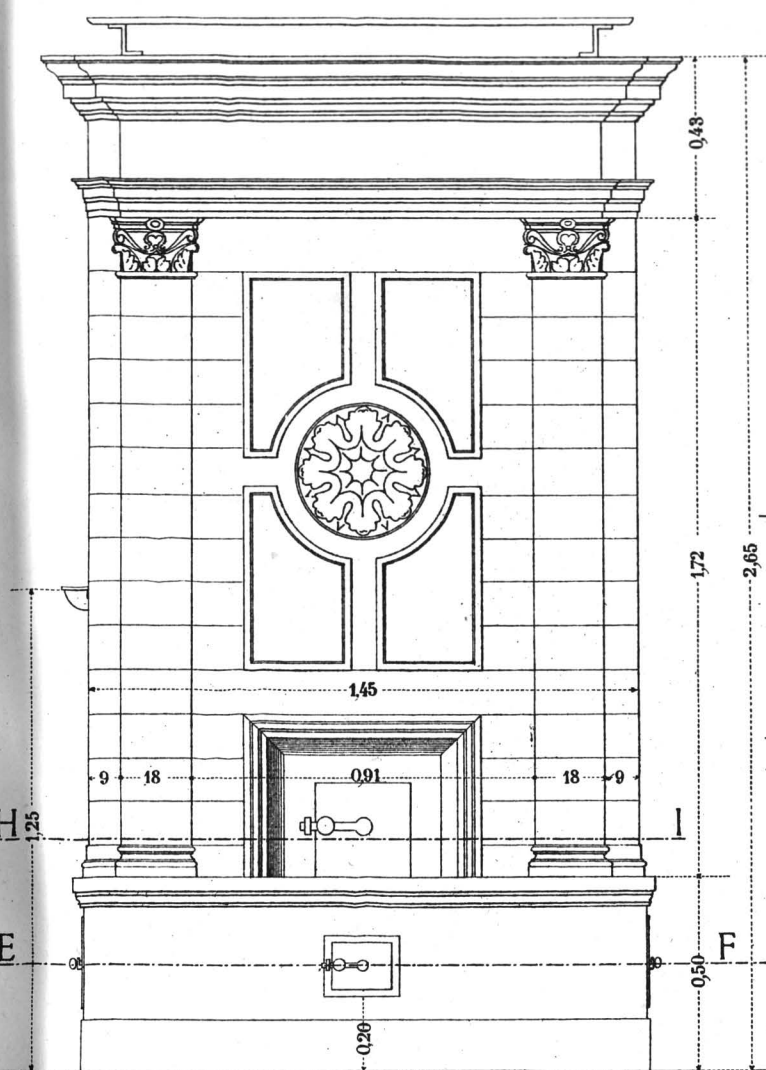
ELEVATIE
