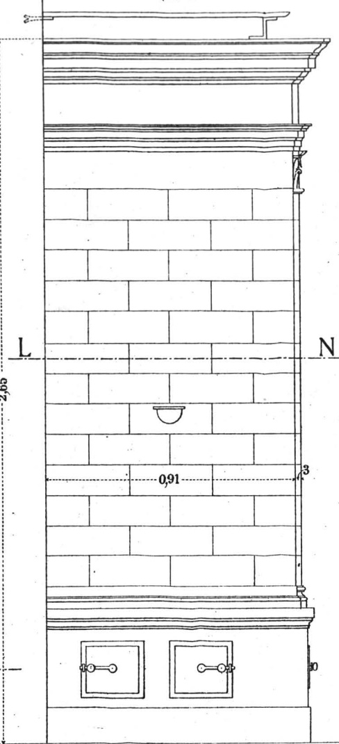
DREAPTA
