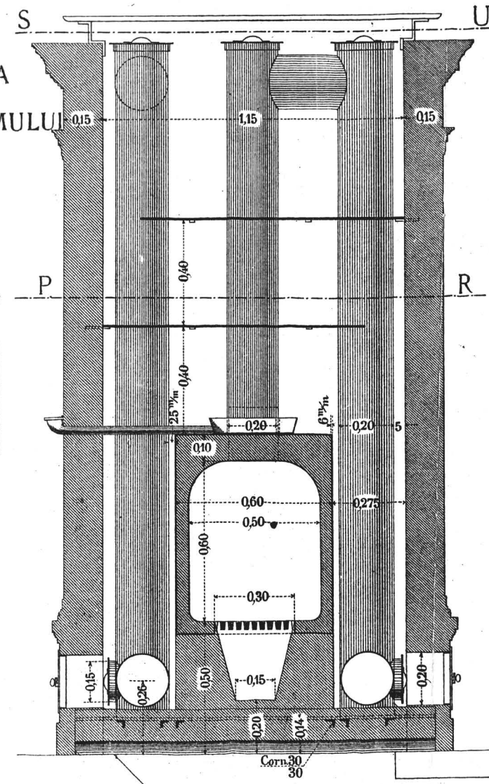
SECTIA AB
