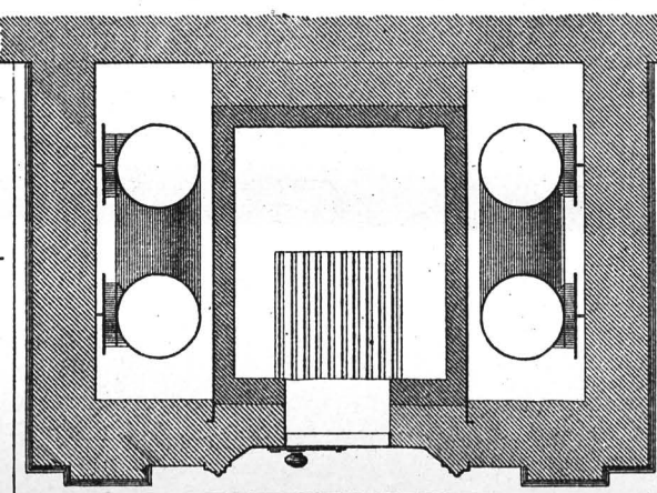
SECTIA HI
