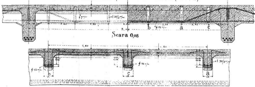
FIG.6 INTOCMIREA DALEI ŞI GRINZII SECUNDARE ( E_x I si II)
