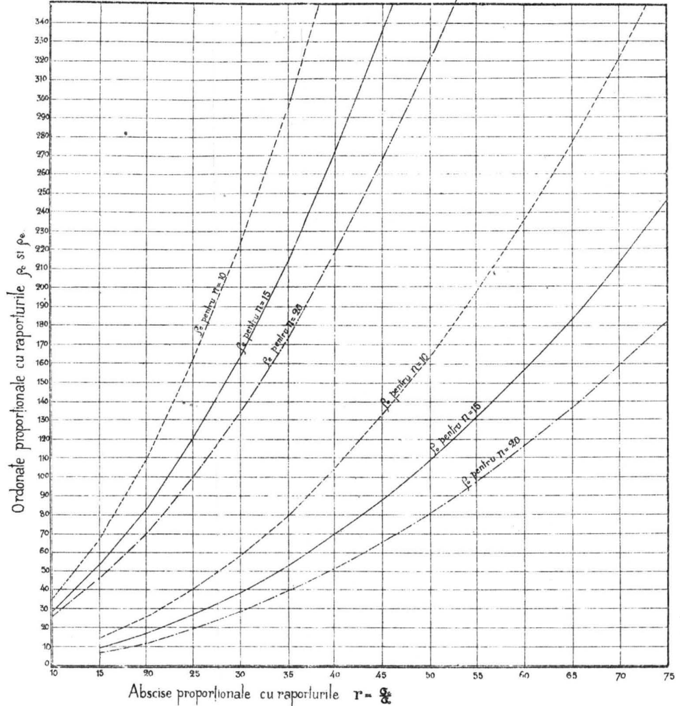
FIG.6 INTOCMIREA DALEI ŞI GRINZII SECUNDARE ( E_x I si II)
