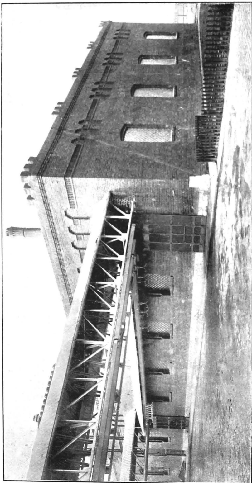
Liniile aeriene de legătură între hale și frigorifere
