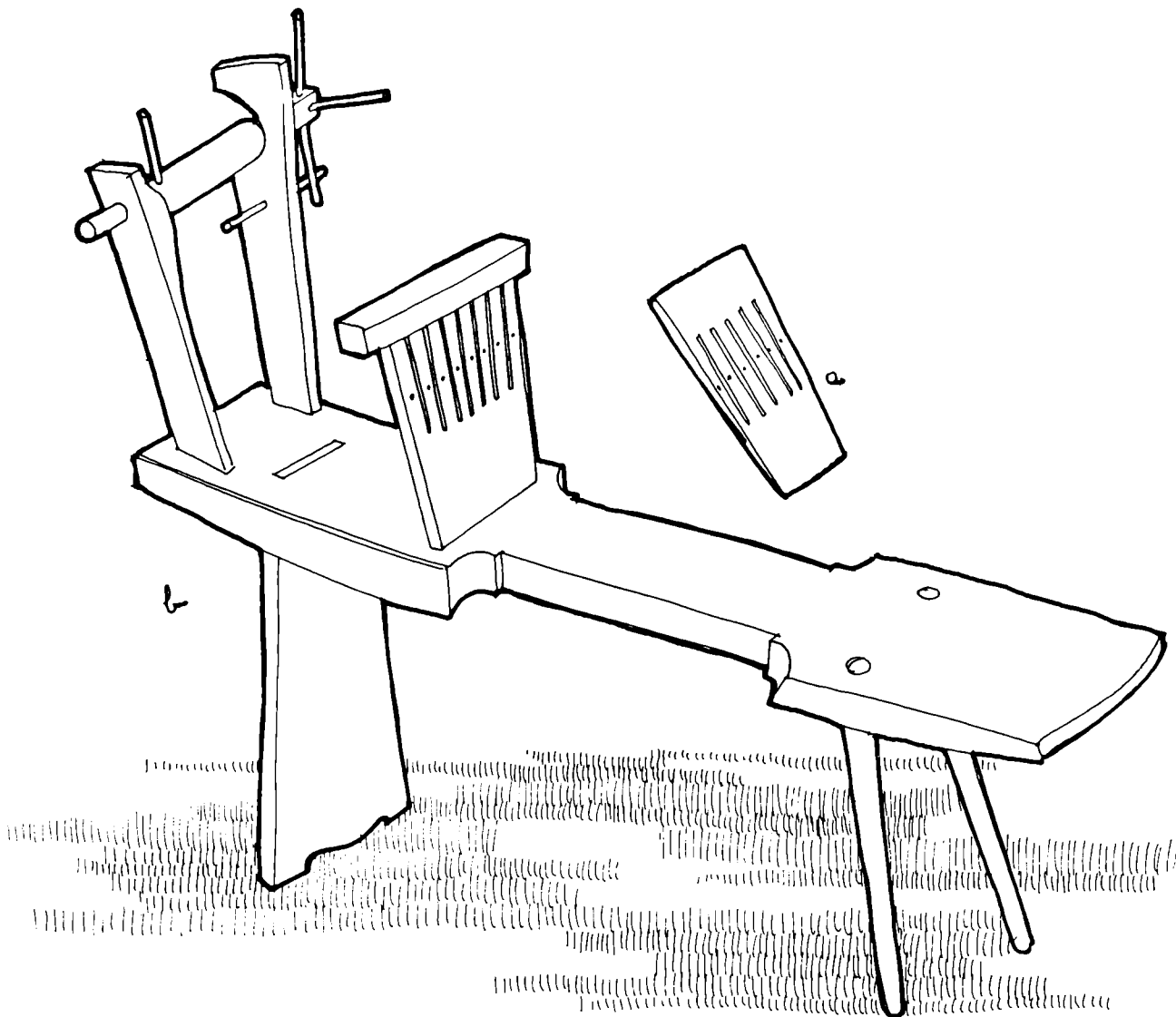
Fig. 1. a — tăbliță pentru țesut; b — război de țesut bete în care tăblița și sulul de urzeală sunt fixate pe un scaun special
