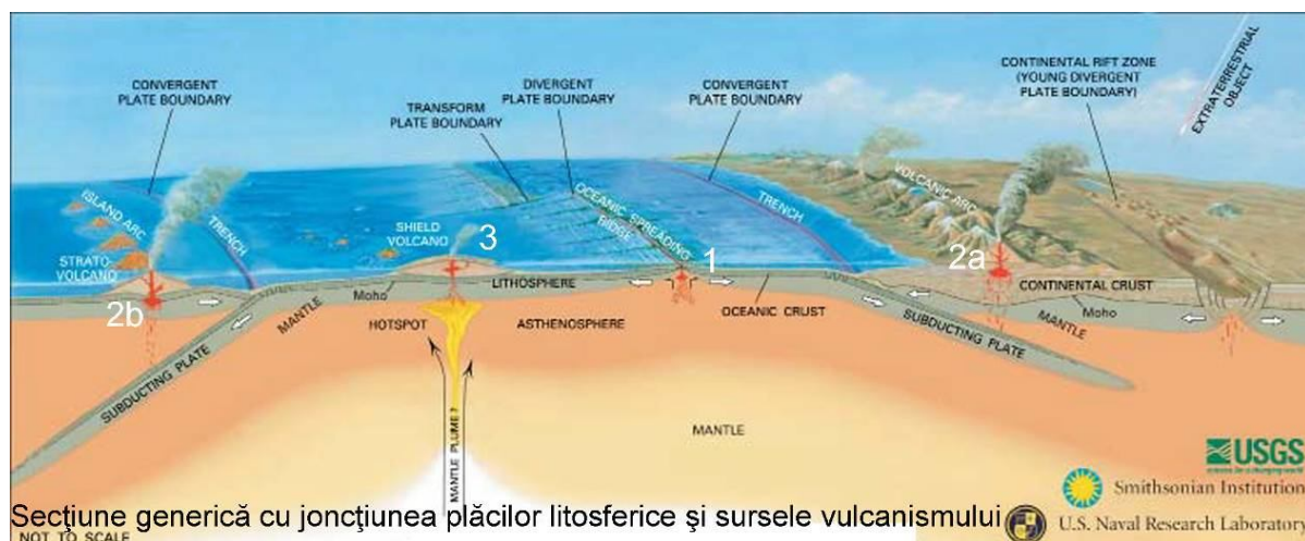
Fig. 1. Secțiune ilustrativă prin crustă/manta cuprinzând contactele generice ale plăcilor litosferice cu tipurile de contacte ale acestora (distensive, convergente) și a punctelor/mecanismelor de generare a vulcanismului:
