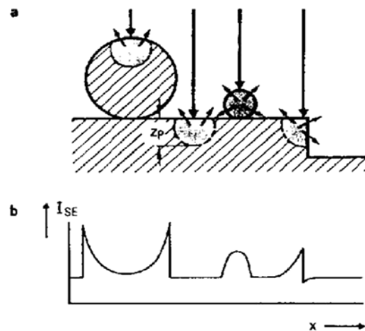
17. ábra. Szekunder elektronjellel különböző objektumokról.
