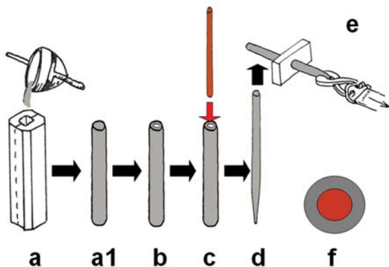
6. ábra. „Bélelt” ezüstdrót készítése: a. ezüstrúd öntése, a1. ezüstrúd, b. kifűrt ezüstrúd, c. vörösréz rúd illesztése az ezüstbe, d. a dróthúzáshoz előkészített, bélelt ezüstrúd, e. dróthúzás, f. a kapott drót keresztmetszete.
