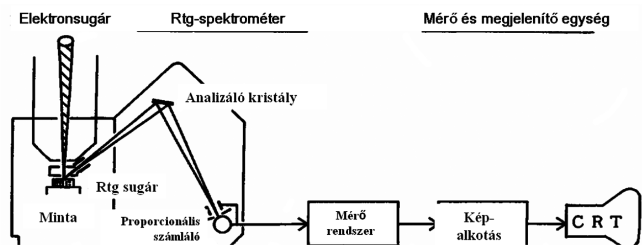
27. ábra. A hullámhosszdiszperzív röntgenspektrométer (WDS) vázolata.
