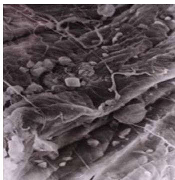
1. kép. Timsós cserzésű bőr a rostok között lerakódott sókristályokkal. Scanning elektronmikroszkópos felvétel.
