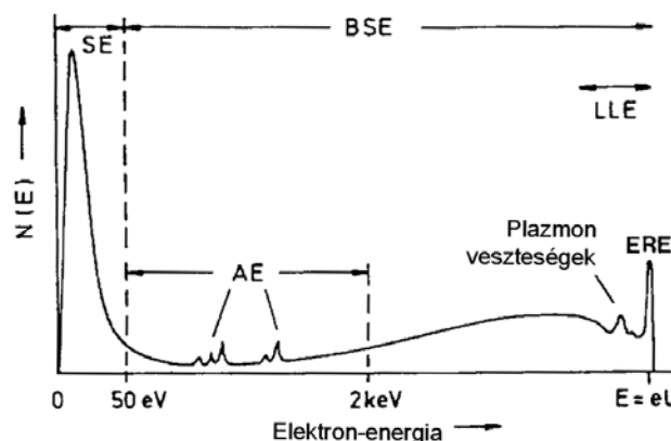
11. ábra. Az emittált elektronok energiaeloszlása.
