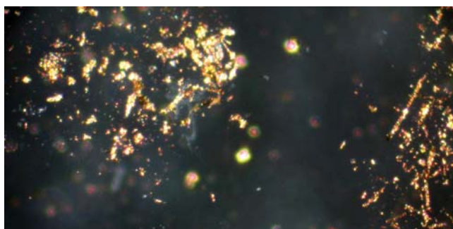
12. kép. A 11. képen látható fonál szalagja: a. salétromsavas megcseppentés után (az ezüst és a réz feloldódott, az arany visszamaradt), b. az oldatban a nátrium-klorid oldat hozzáadása után fehér csapadék keletkezik (ezüst-klorid).
