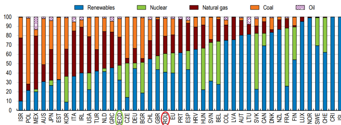
Figura 1: Producerea de energie electrică după sursa de energie
