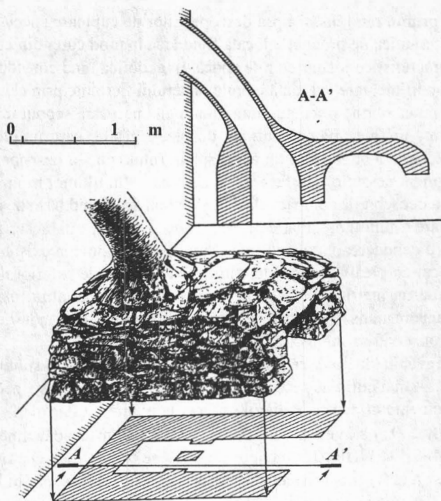
Fig. 3. Reconstituirea ipotetică a cuptorului locuinței nr. 1.
