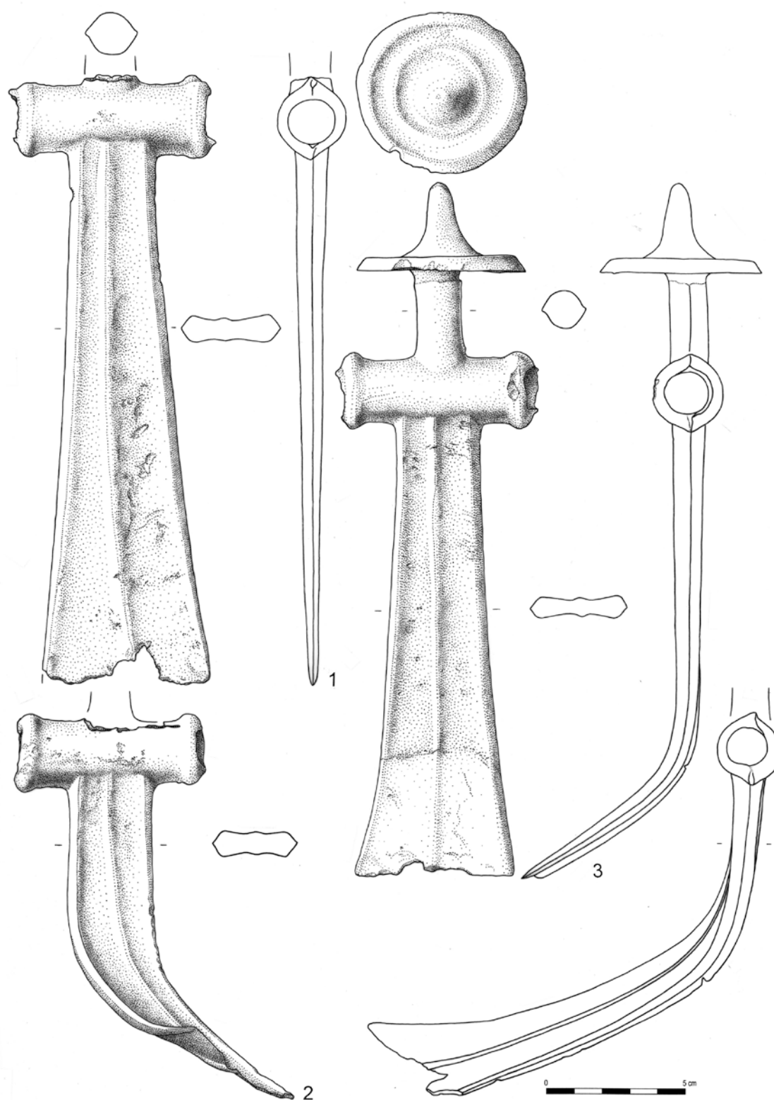
Pl. 43. Lăschia. Depozit de bronzuri.
