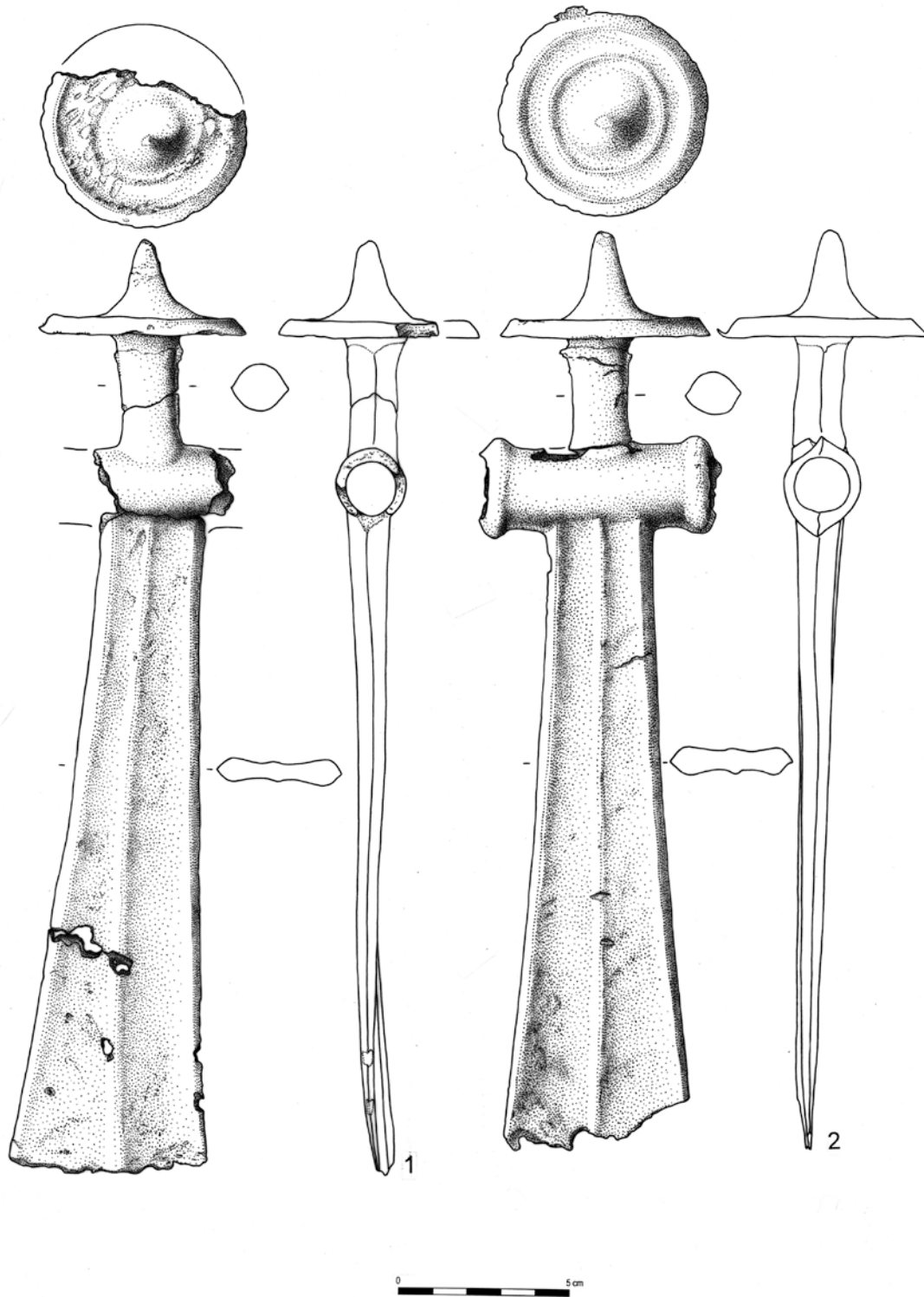
Pl. 39. Lăschia. Depozit de bronzuri.
