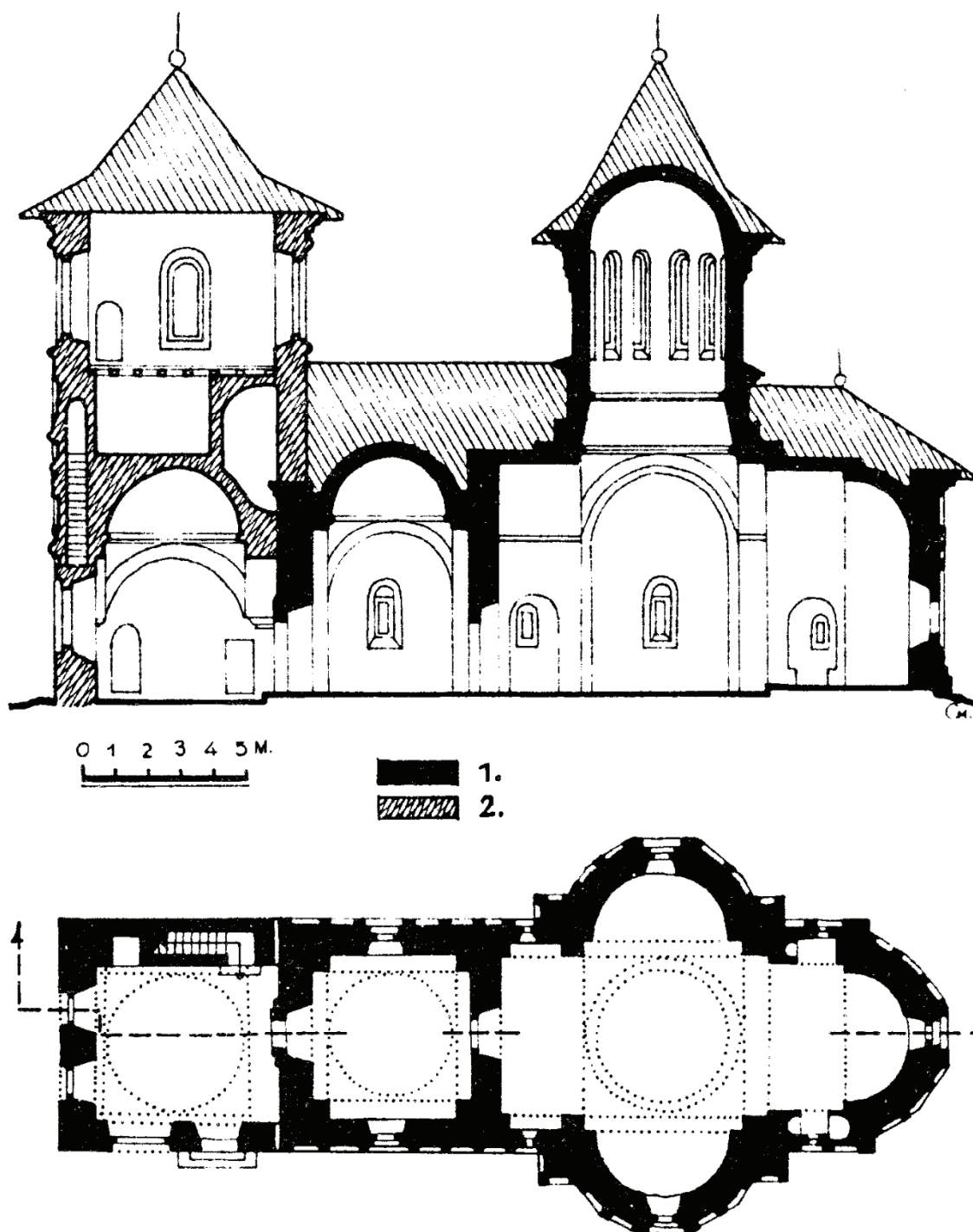
Fig. 5. Biserica mănăstirii Jitianu, jud. Dolj. Plan și secțiune. 1. 1656; 2. 1701. (Moisescu, Arhitectura , vol. II, p. 98, fig. 119)
