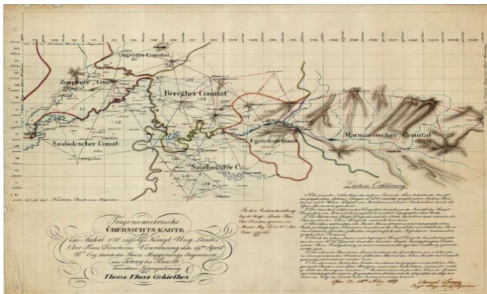
Fig. 4. Extinderea rețelei de triangulație în zona Tisei superioare în anul 1836.
