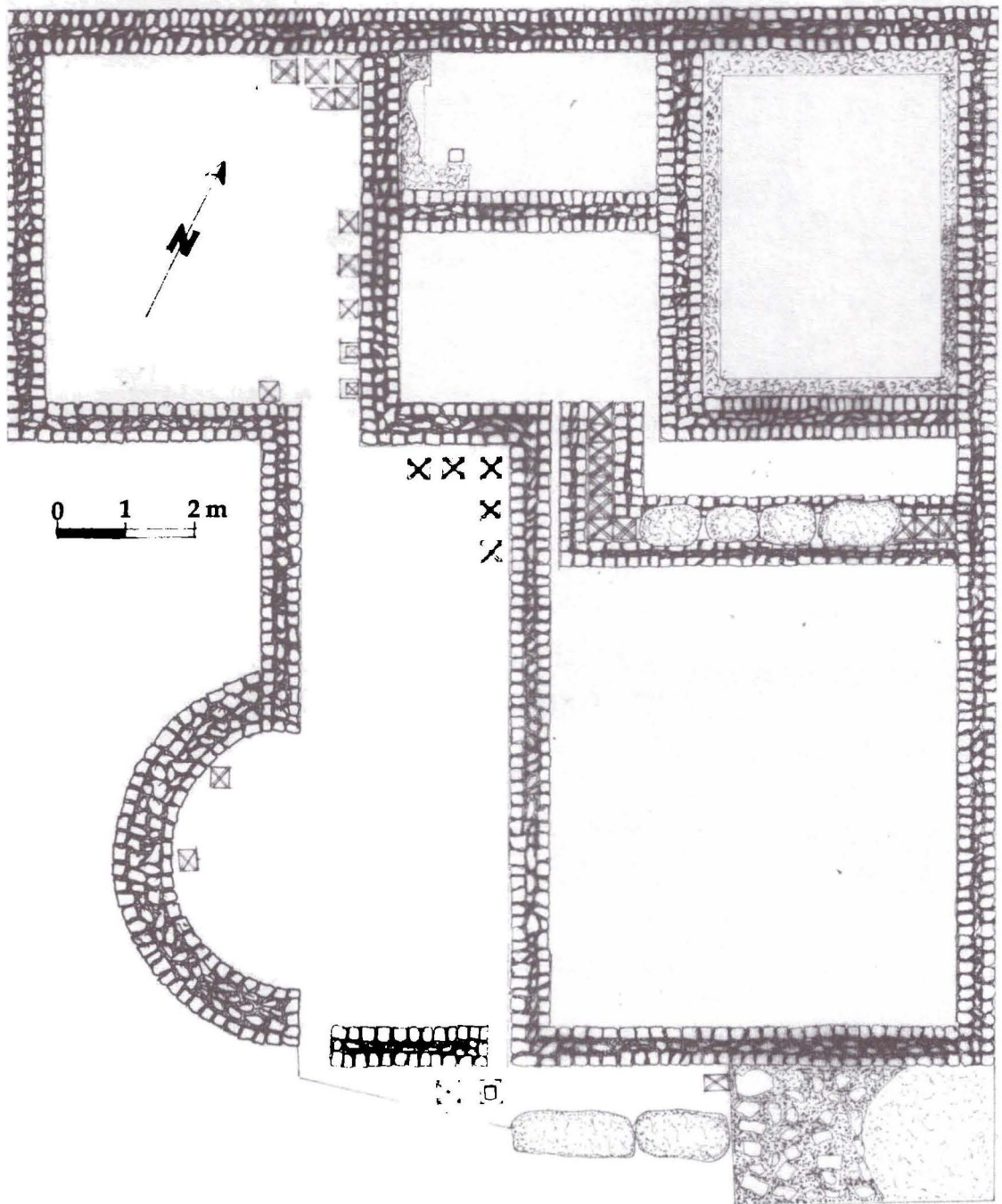
Pl. IV. Zăvoi. Planul cercetărilor efectuate în anul 2009 la Domus.
