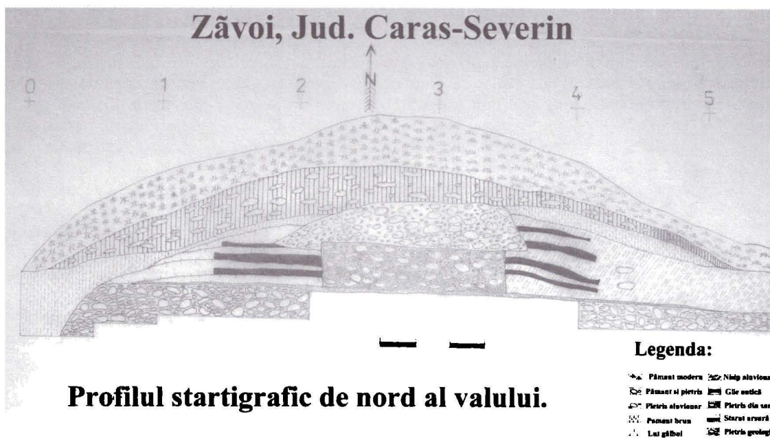
Pl. II. Zăvoi. Profilul stratigrafic de nord al valului.
