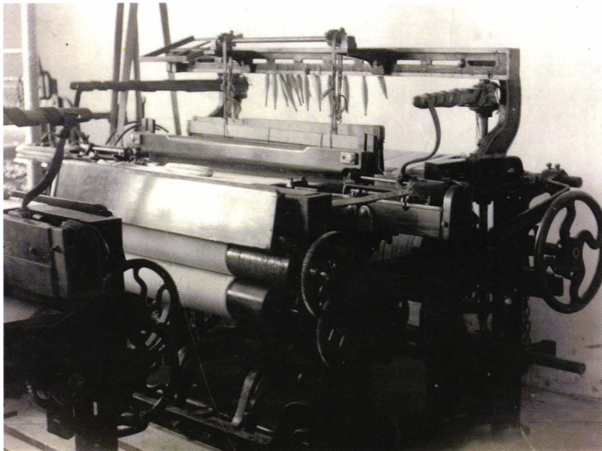
Război mecanic, țesătoria fraților Ionescu
