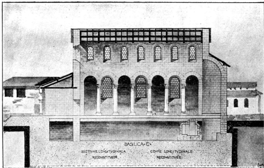
Fig. 33 (archit. Cegăneanu).
