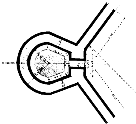
Fig. 12. Turnul de colț dela NV (arhit. Fakler).
