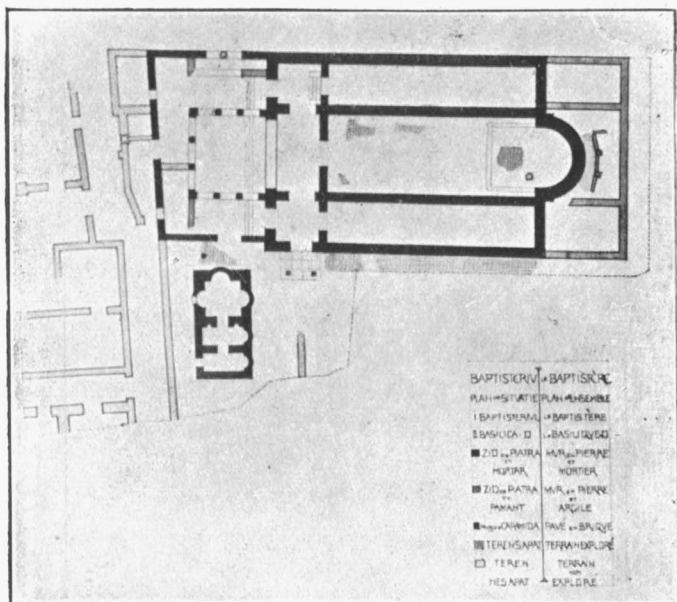
Fig. 20. Planul orizontal al basilicii de marmoră, cu baptisteriul și clădirile târzii înconjurătoare (archit. Cegăneanu).
