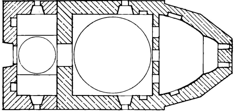
Fig. 5. -- Mănăstirea Frăsinei. Planul bisericii vechi.
