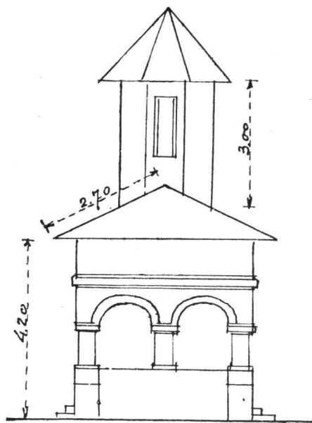
Fig. 5. Schitul Bunea. Fațada de Vest.
