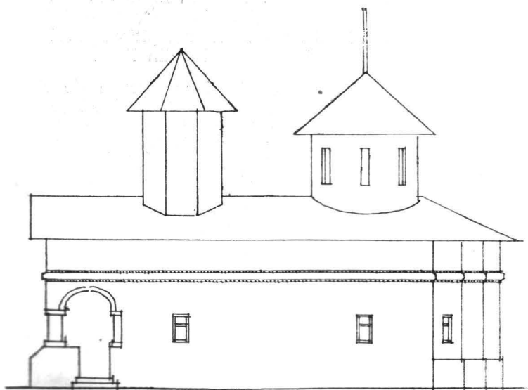
Fig. 4. — Schitul Bunea. Fațada de Sud.
