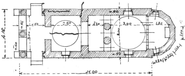
Fig. 3. — Schitul Bunea. Planul bisericii.
