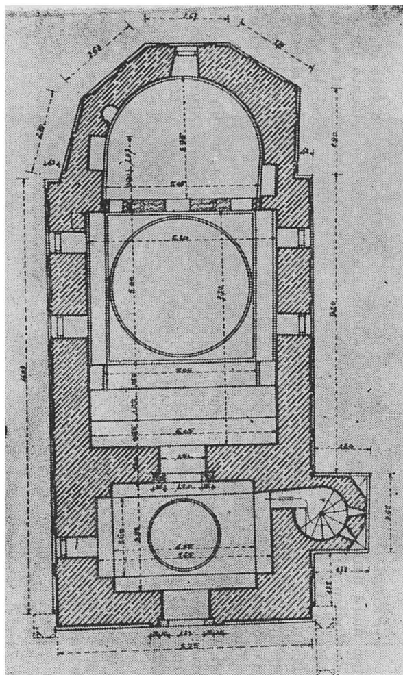
Planurile bisericilor Strehaia (1) și Gherghița (2) (după BCMI, 1936, pl. LVII și XVIII).
