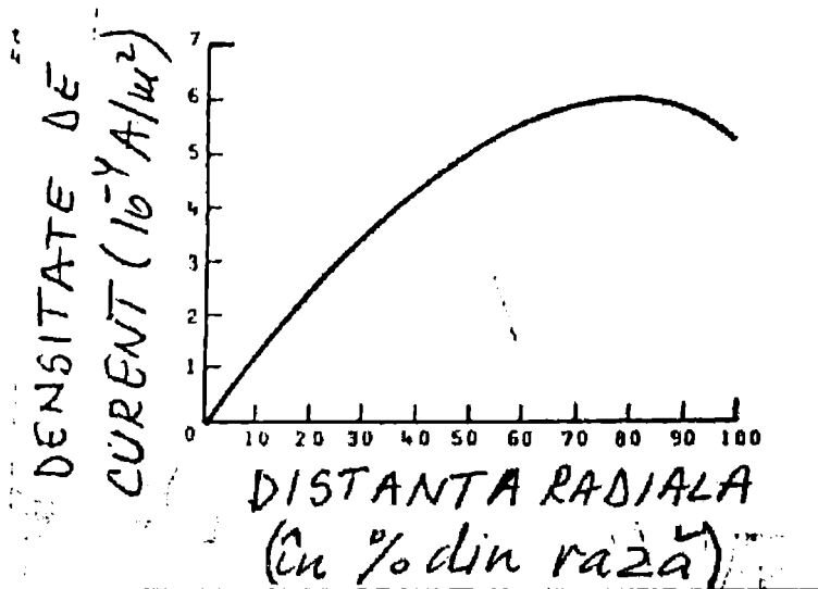
Fig. 9.5. Curentul total din inima pământului în funcție de distanța de la centrul pământului, în % din raza pământului.
