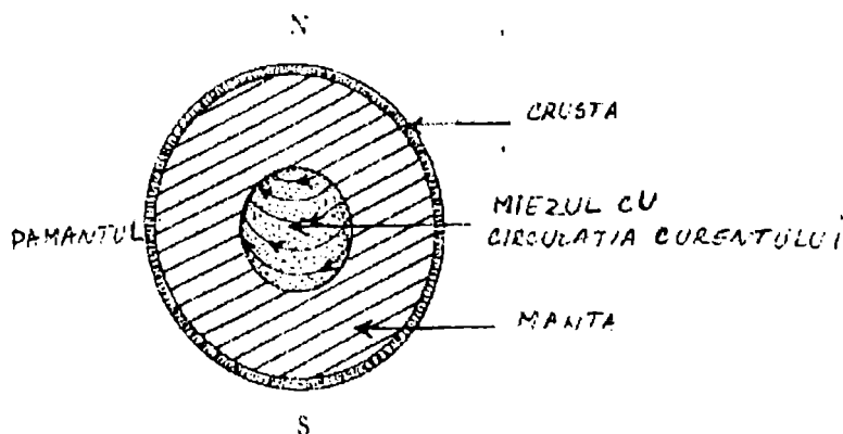
Fig. 9.4. Circulația curentului în interiorul pământului, produce câmpul magnetic al pământului.
