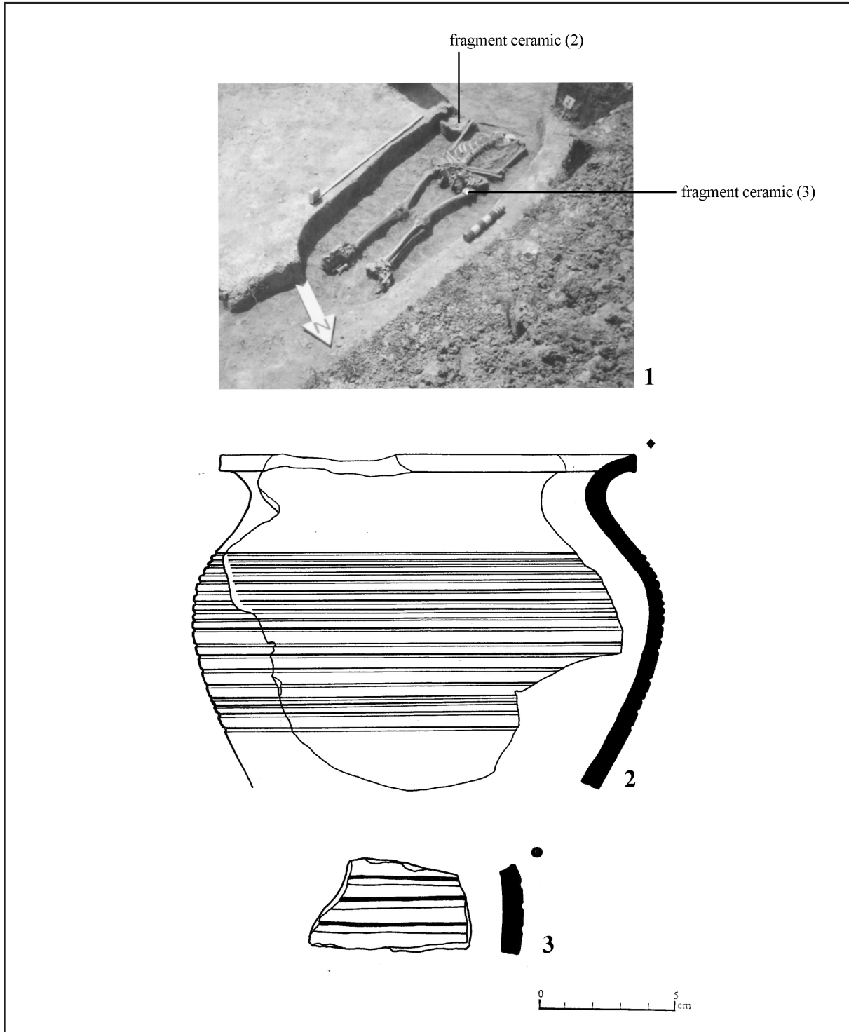
Fig. 7. Zalău-Valea Răchișorii/Pálvár. Mormântul M. 2/2001/(după Băcueț-Crișan 2015).
