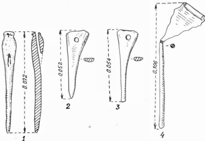
Рис. 7. — Трушешти — Мовила в долине Жижкии. Бронзовые и костяные проколки позднебелопотоцкой культуры.
