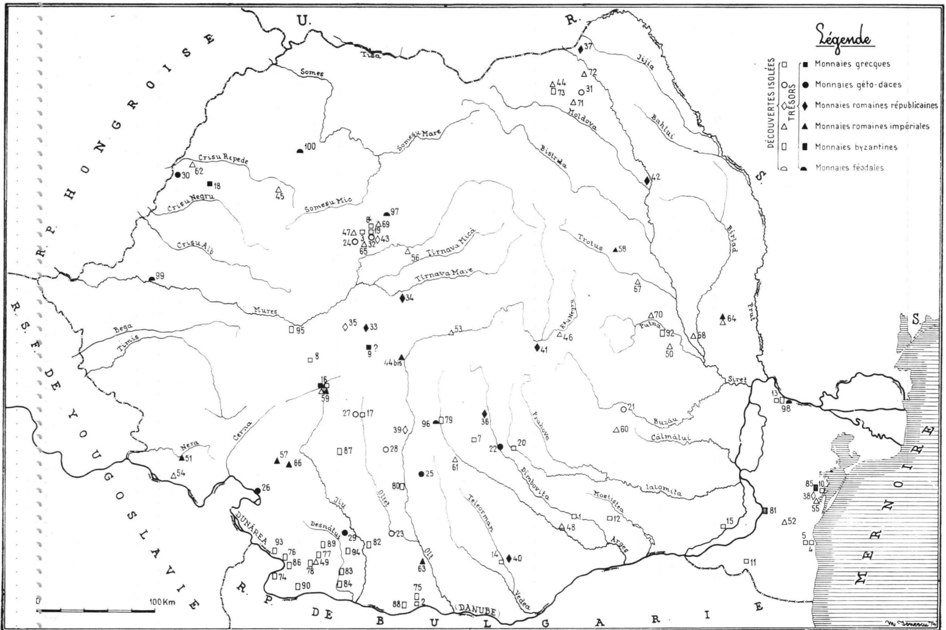
Fig. 2. La carte des découvertes de monnaies antiques et byzantines dans la République Socialiste de Roumanie(1974).
