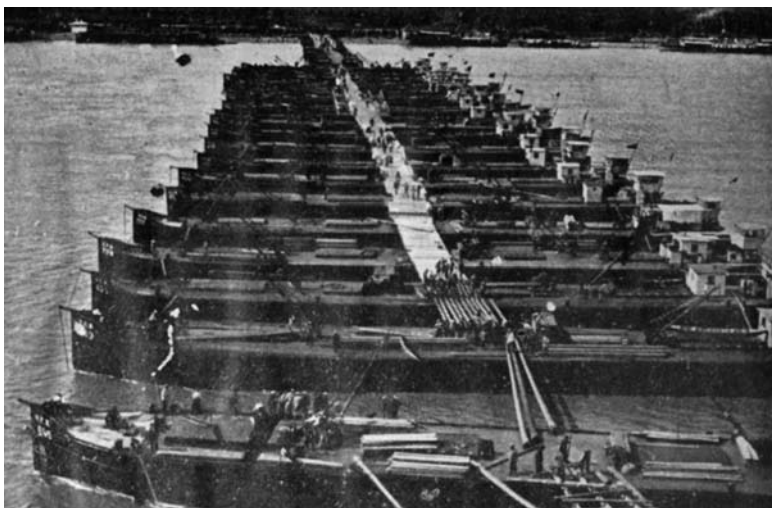
Construcția podului de la Turnu Măgurele
