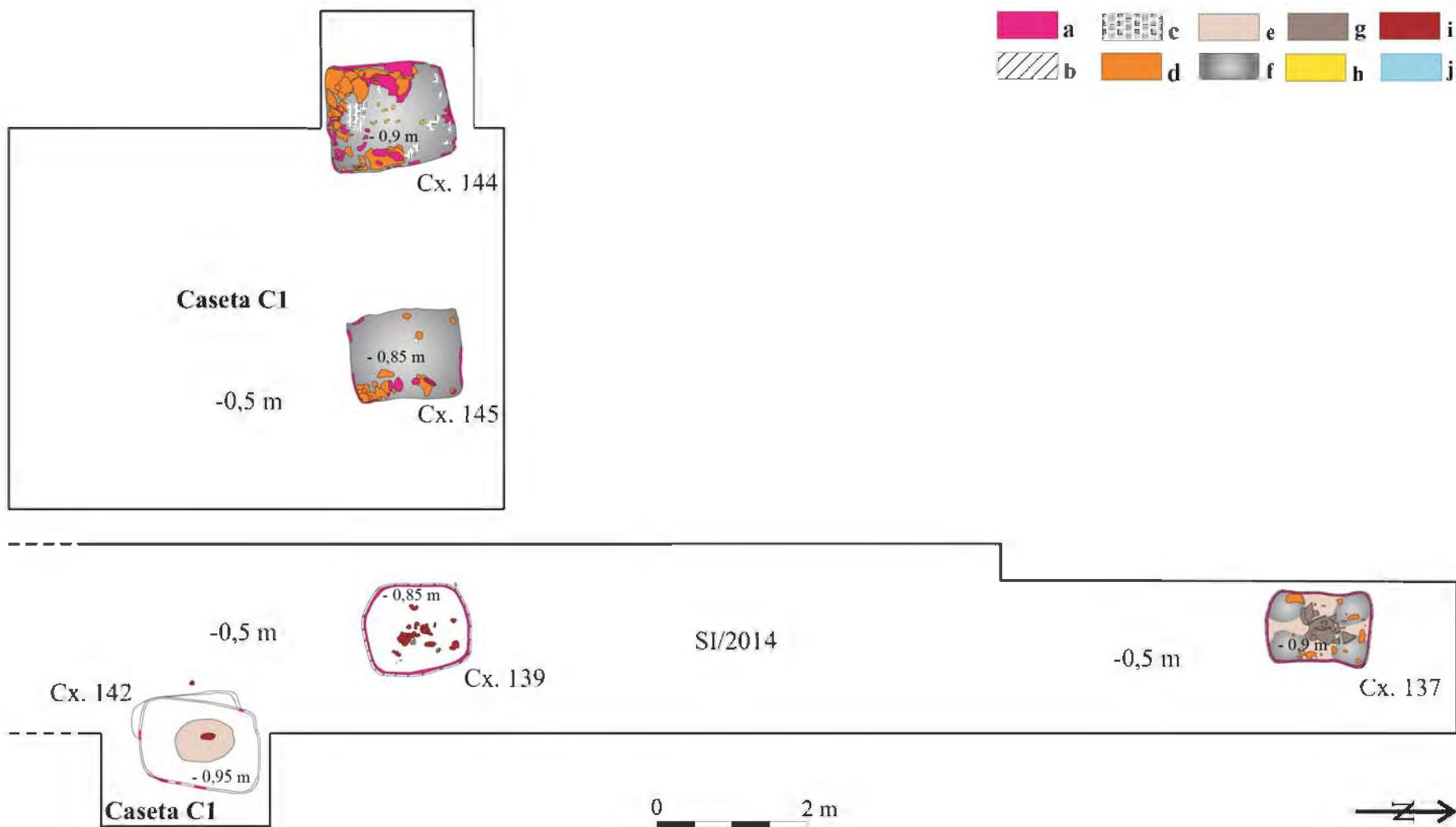
Fig. 3: Desen al secțiunii SI/2014 și al casetelor C1 și C4 din 2014. Legenda: a- perete lutuit și ars; b- pământ ars (în exteriorul gropii); c- lemn carbonizat; d- lipitură prăbușită din pereții gropii, amestecată cu cărbune; e- nisip ars la roșu; f- cărbune amestecat cu cenușă; g- fragmente ceramice; h- oase arse; i- material metalurgic; j = fragmente silex.
