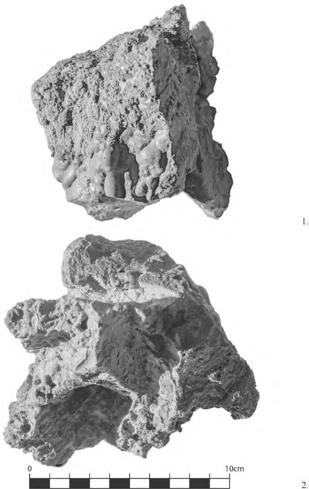
Fig. 12: Zgură de cuptor descoperită în complexul 158/159, 630 gr. Fotografii ce prezintă partea exterioară a zgurii ce a fost lipită de peretele cuptorului (1) și partea interioară ce prezintă urmele lăsate de cărbune (2).
