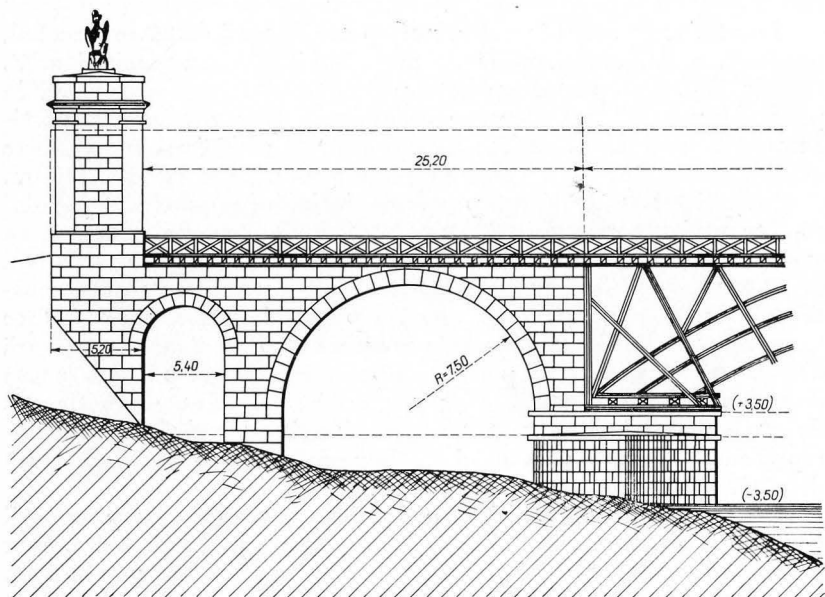
II. Capătul nordic al podului lui Traian (reconstituire după ing. Edgard Duperrex)
