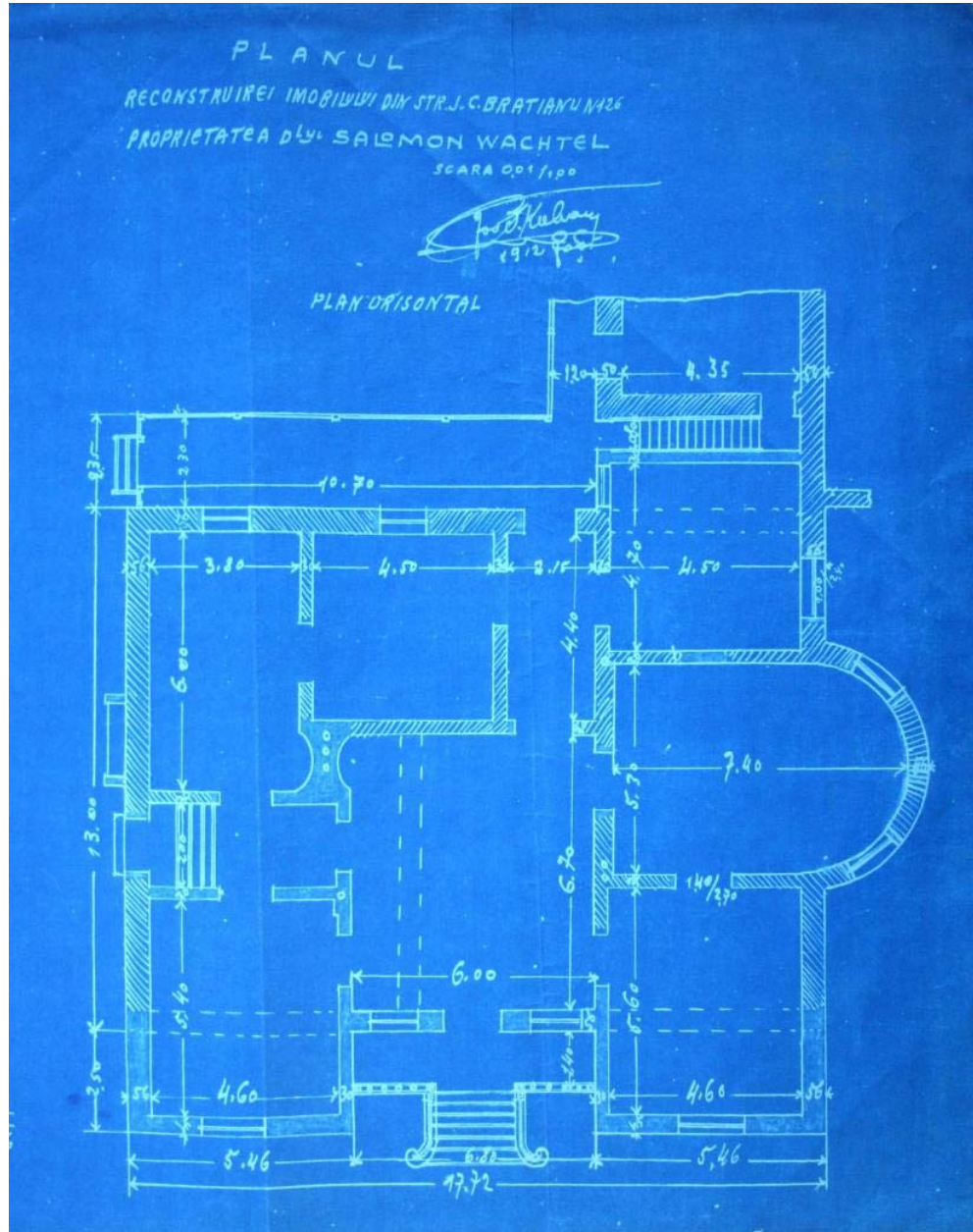
Fig. 44 – Str. I.C. Brătianu Planul casei Wachtel (1912)
