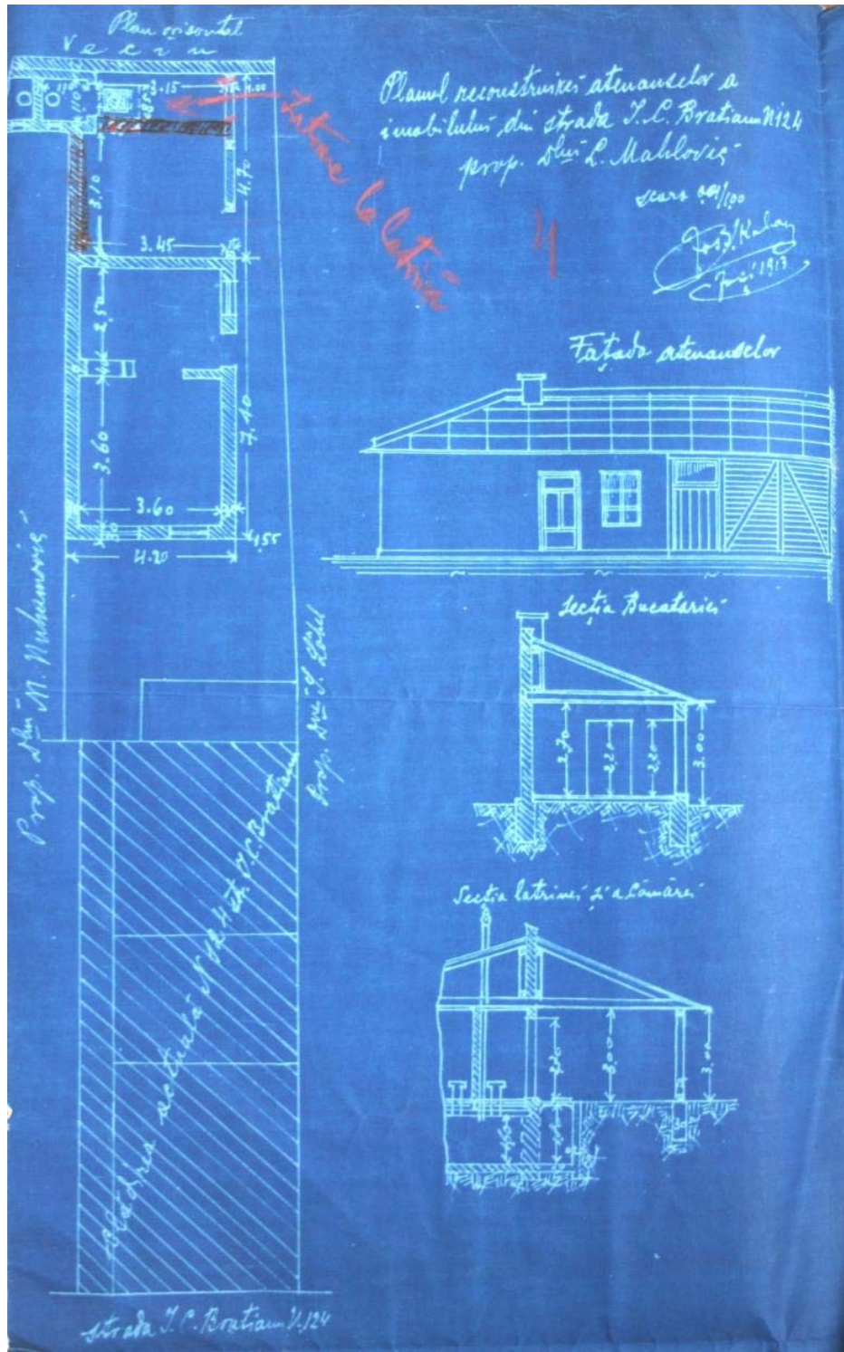
Fig. 40 – Str. I.C. Brătianu nr 124 Planul reconstruirii atenei proprietății Mahlovici (1913)
