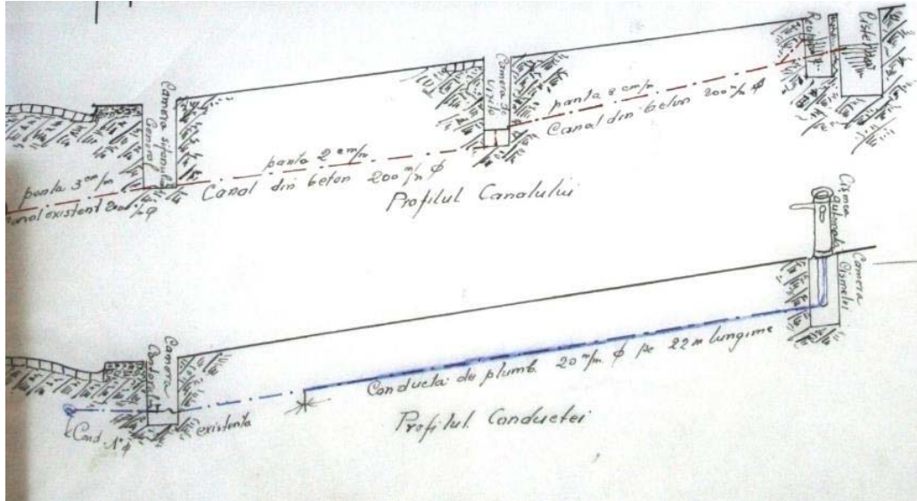
Fig. 35 – Str. Universității nr. 12 (dreapta). Amenajarea instalației de canalizare
