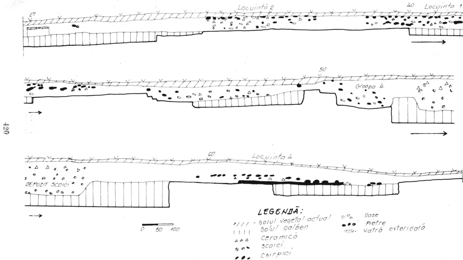
PL. I — PROFILUL SECȚIUNII PL. I — LE PROFIL DE LA TRANCHÉE. TAF. I QUERSCHNITT
