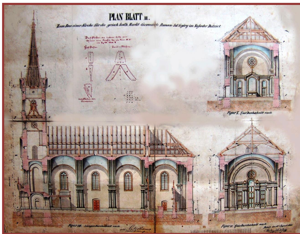
Planul Bisericii „Sfântul Nicolae” (Fotografie din colecția artistului Maxim Dumitraș)
