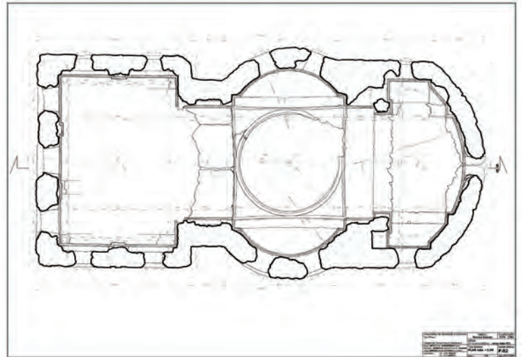
Fig. 10. Planul ruinei bisericii Mănăstirii Giulești. Relevu redesenat și completat de stud.arh. I. Butu, 2009
