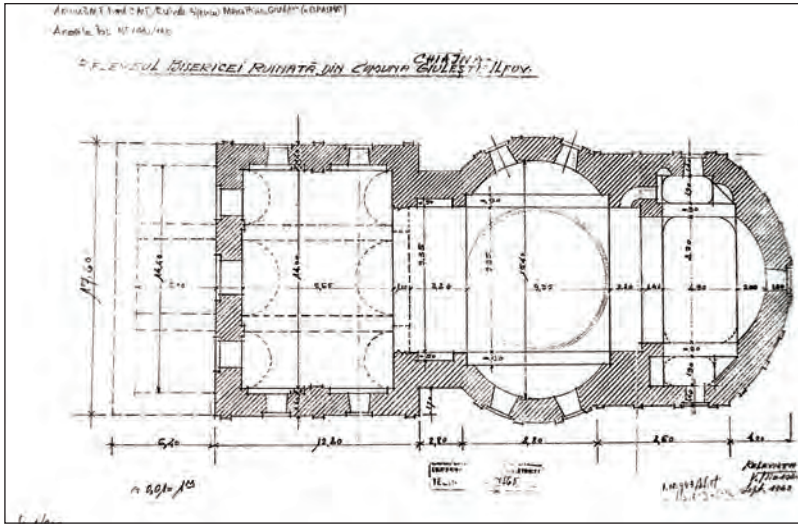
Fig. 9. Planul ruinei bisericii Mănăstirii Giulești. Relevu arh. V. Moisescu, 1946, Fondul CMI, Arh. INP
