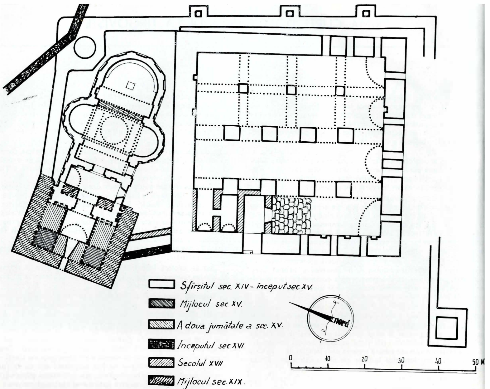
Fig. 1. Prima Curte domnească din Tîrgoviște. Plan la nivelul beciurilor.
