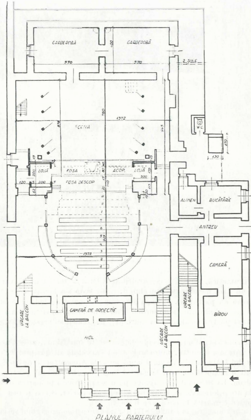
Fig. 4. — Teatrul din Oravița. Planul parterului.
