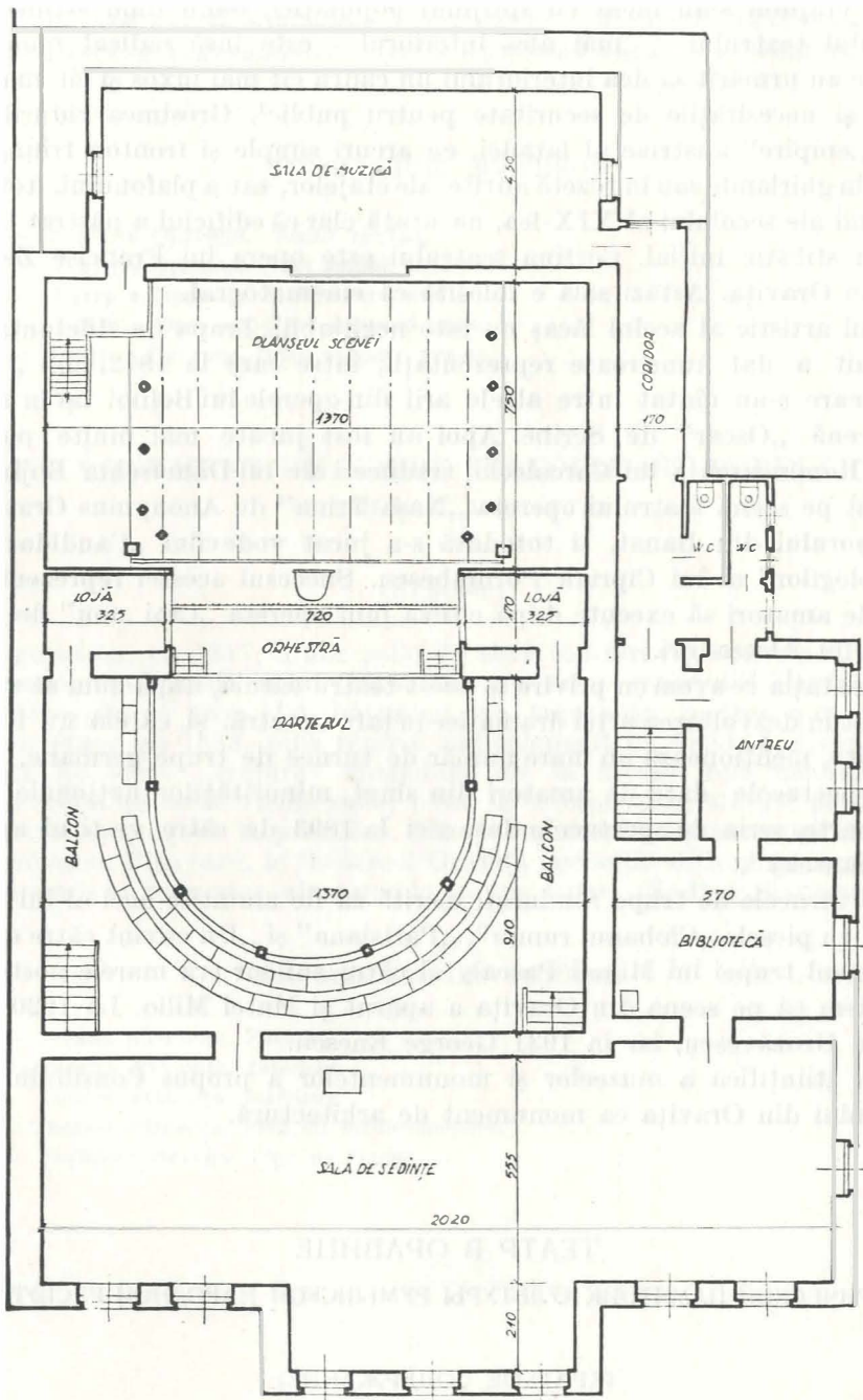
PLANUL ETAJULUI
