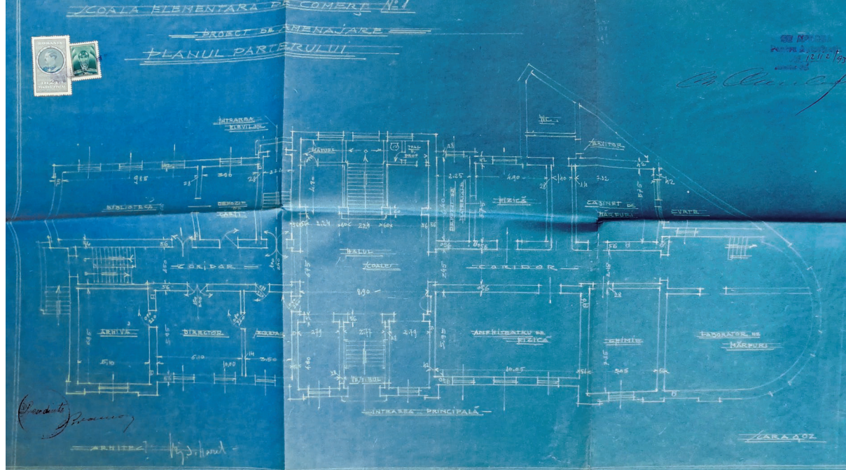
Fig. 9 Etapa 1929-1934 - Planul parterului cu extinderea cu volumul semicircular Sursa: Arhiva PMB, Fond II Negru, Dosar 712/1929
