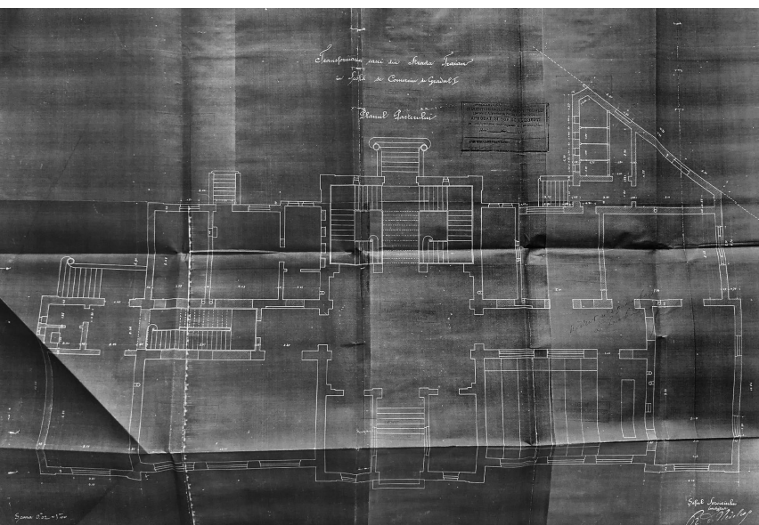
Fig. 3 Etapa 1895 - Plan parter Sursa: ANR-DMB, Fond PMB Serviciul Tehnic, Dosar 1205/1895
