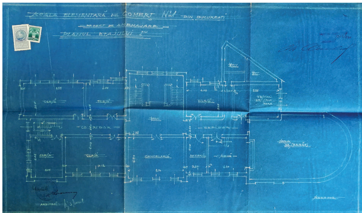
Fig. 10 Etapa 1929-1934 - Planul etajului 1 cu extinderea cu volumul semicircular Sursa: Arhiva PMB, Fond II Negru, Dosar 712/1929
