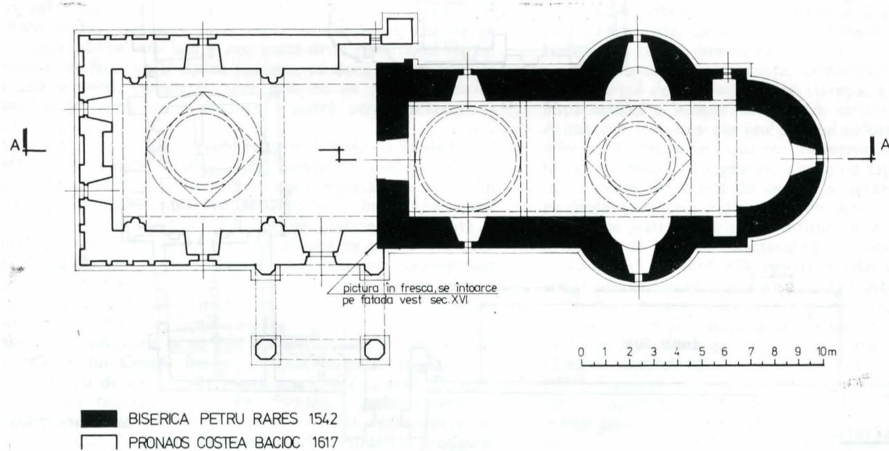
Biserică Plan 1:100
