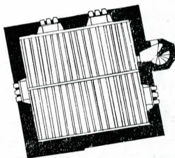
PLAN ETAJ II
