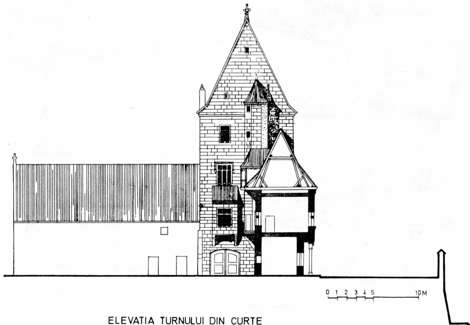
Fig. 5. — Primăria Veche. Elevația turnului văzută din curte.
