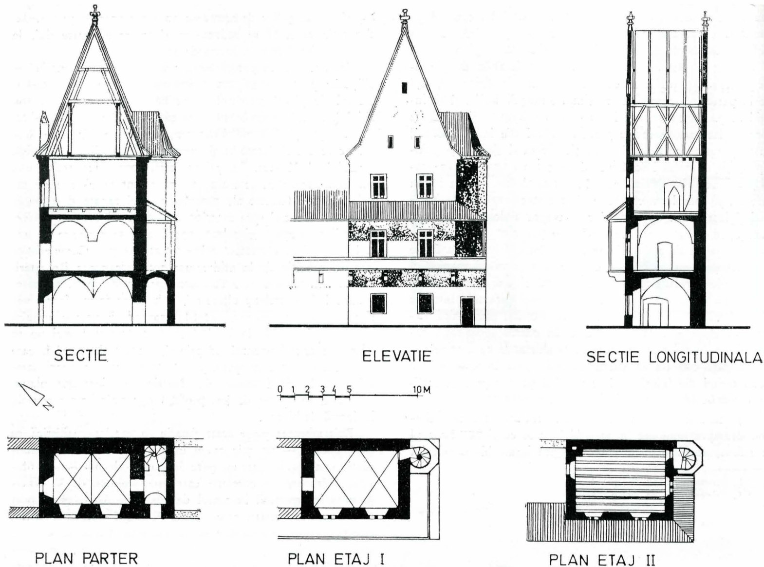
Fig. 7. — Casa Haller. Fațada, planuri și secții prin turn.
