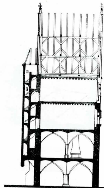
SECȚIE NORD-SUD
