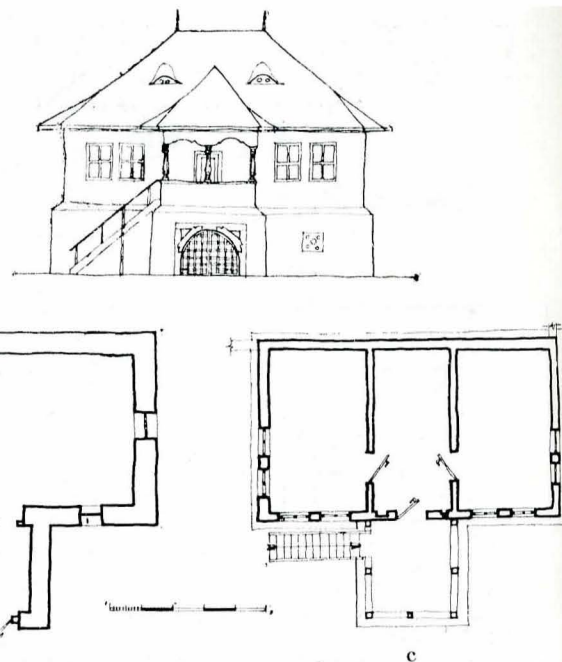
Fig. 14. Casă la Seciu datînd din a doua jumătate a secolului al XVIII-lea extinsă și transformată spre mijlocul secolului al XIX-lea în conac boieresc (reconstituirea nucleului datînd din secolul al XVIII-lea): a — fațada principală, b — planul beciului, c — planul nivelului de locuire.
