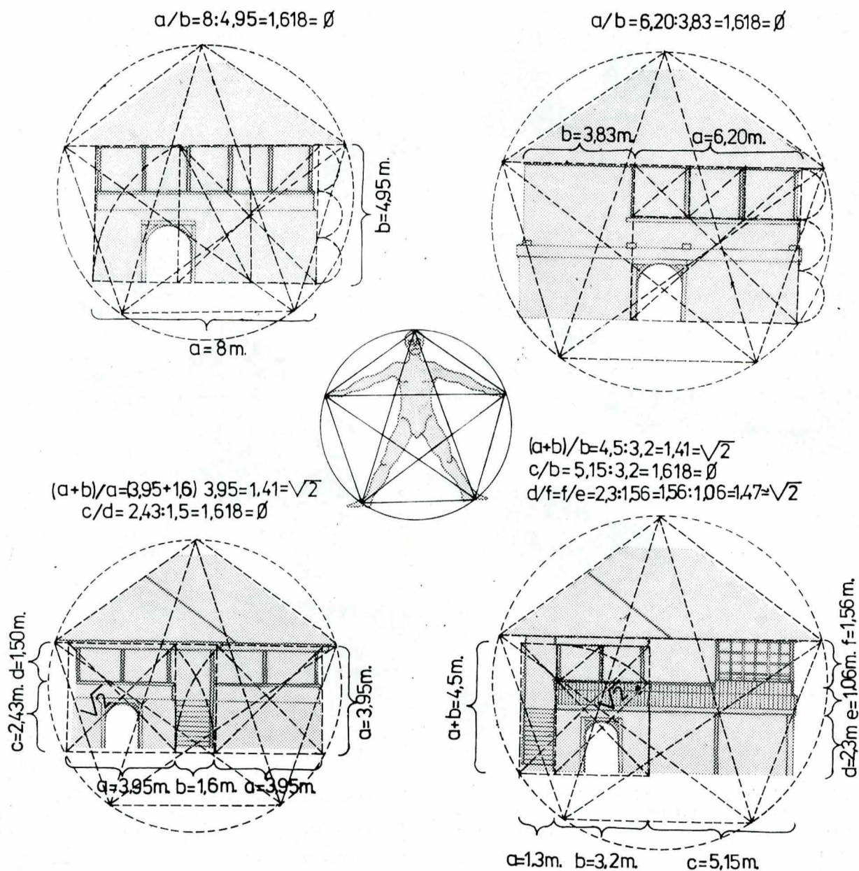
Fig. 20. Trasee reguloare utilizate la proporționarea fațadelor locuințelor sătești din zona Văii Teleajenului:
