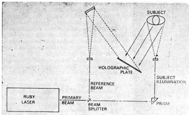
Fig. 3. — Schema aranjamentului componentelor în aparatura holografică
