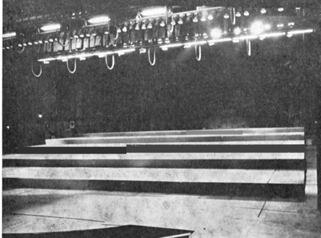
Instalația de iluminare a scenei, complet automatizată
