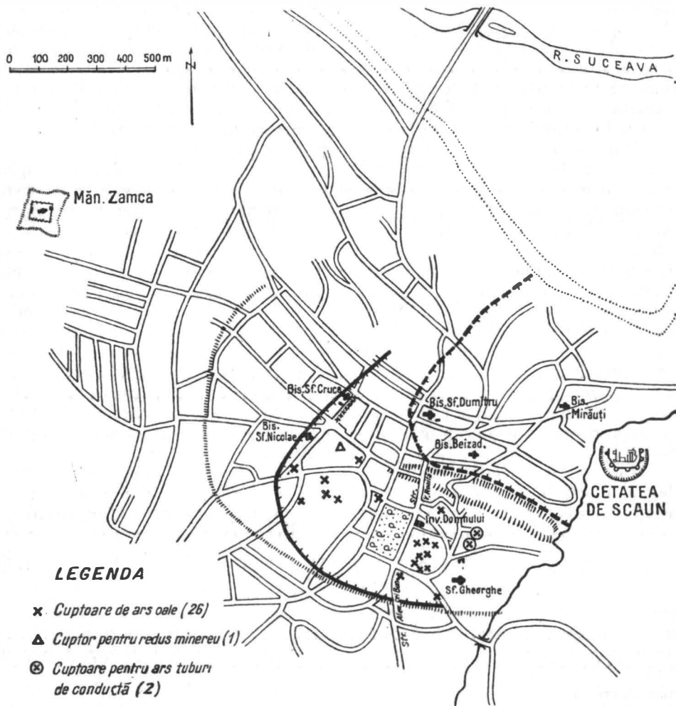
Fig. 1. — Suceava. Colțul sud-estic al parcului, cu amplasarea cuptoarelor de ars oale din sec. XV—XVI.
