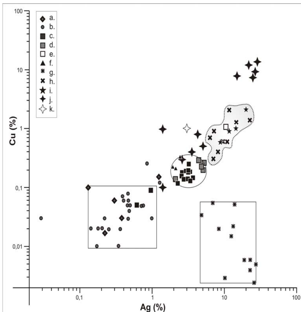
Fig. 1. Raportul dintre procentele de argint și cupru din mai multe monede și brățări de aur (după V. Cojocaru, B. Constantinescu, I. Ștefănescu, C. M. Petolescu, Journal of Radioanalytical and Nuclear Chemistry 246, 1, 2000, p. 188-189, fig. 2 și 4, cu adăugiri). În legendă: a - aurei republicani; b - aurei imperiali; c - monede koson cu monogramă complexă; d - monede koson cu monogramă simplă; e - monede koson fără monogramă; f - stateri postumi Lysimachos; g - probe de aur nativ (România); h - brățările spiralice nr. 1-9 (valori după E. O.-T. și B. C.); i - brățările spiralice nr. 1-4 (valori după B. D.-L.); j - monedele, și k - colanul din tezaurul de la Saint-Louis Basel (după A. Furger-Gunti).
